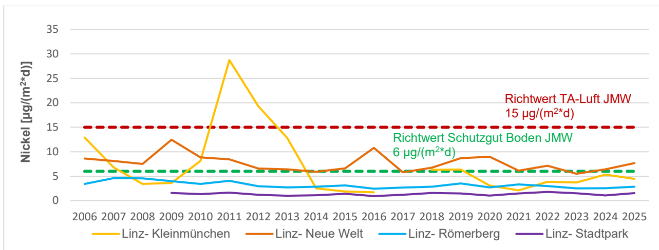
Abbildung 32: Nickel im JMW im Jahrestrend 2006 – 2025
