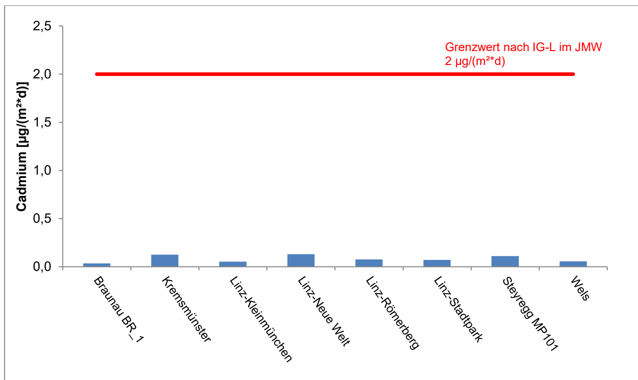
Abbildung 9: Cadmium im JMW der Oö. Messstellen 2025
