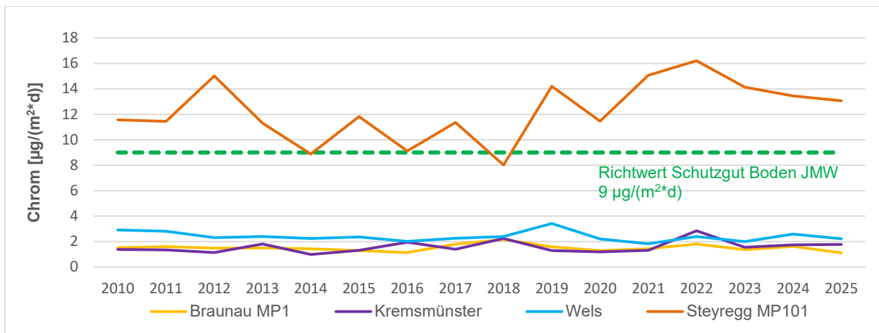
Abbildung 23: Chrom im JMW im Jahrestrend 2010 – 2025
