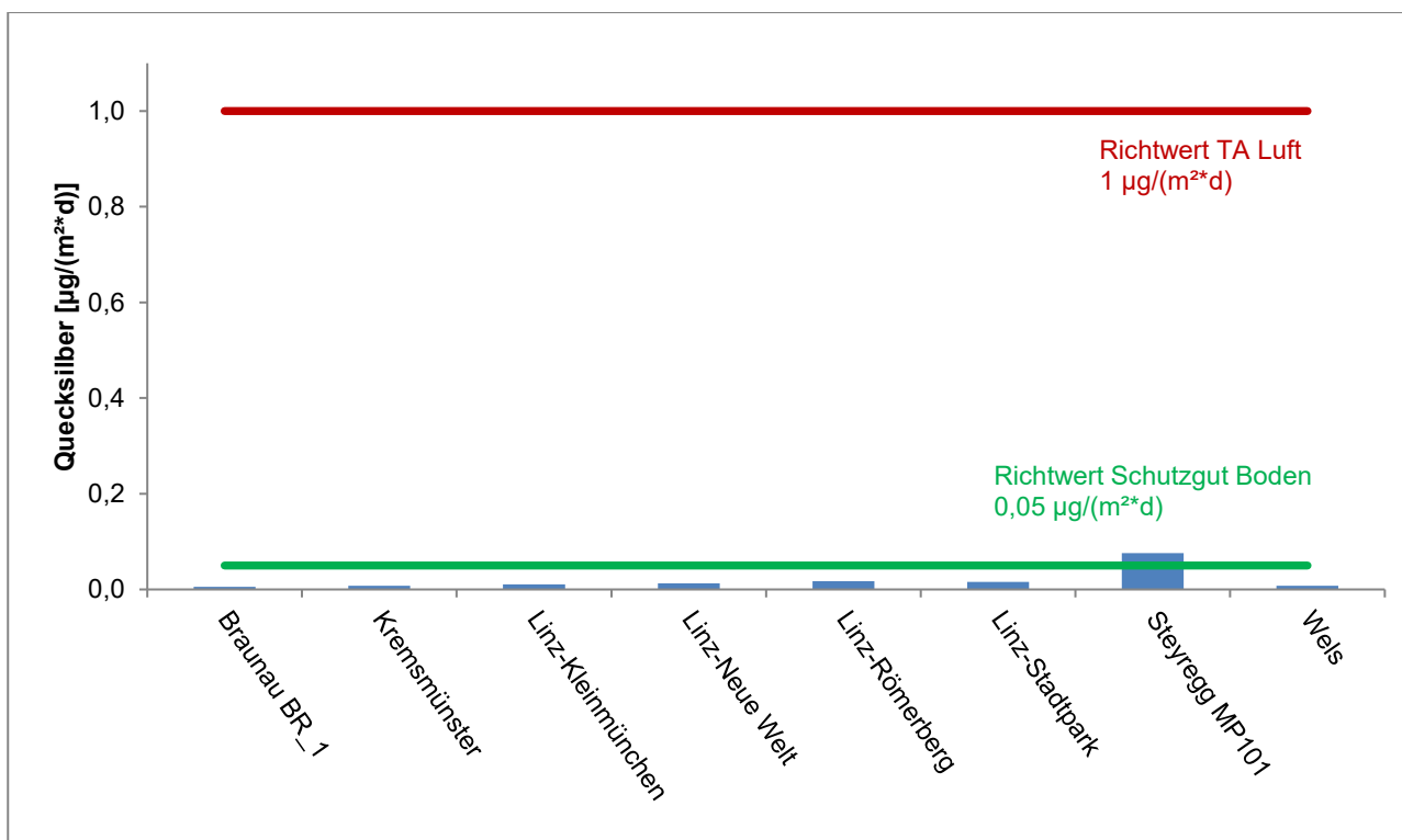
Abbildung 16: Quecksilber im JMW der Oö. Messstellen 2025
