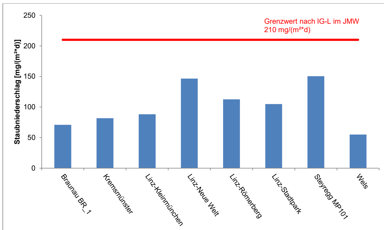
Abbildung 7: Staubniederschlag im JMW der Oö. Messstellen 2025
