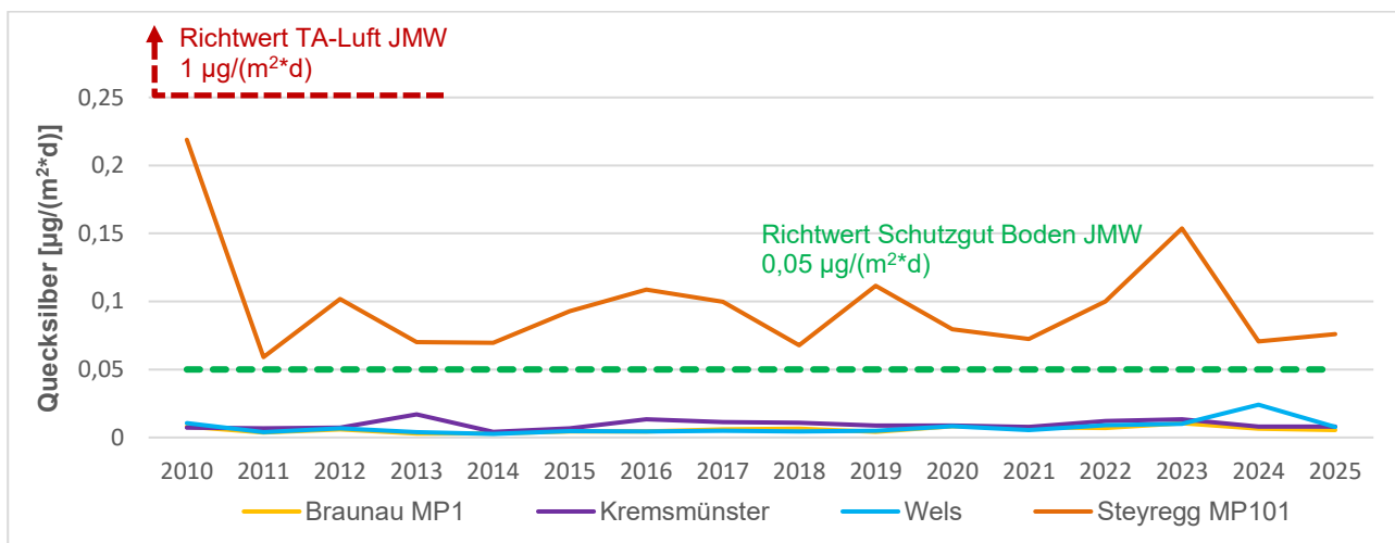
Abbildung 27: Quecksilber im JMW im Jahrestrend 2010 – 2025
