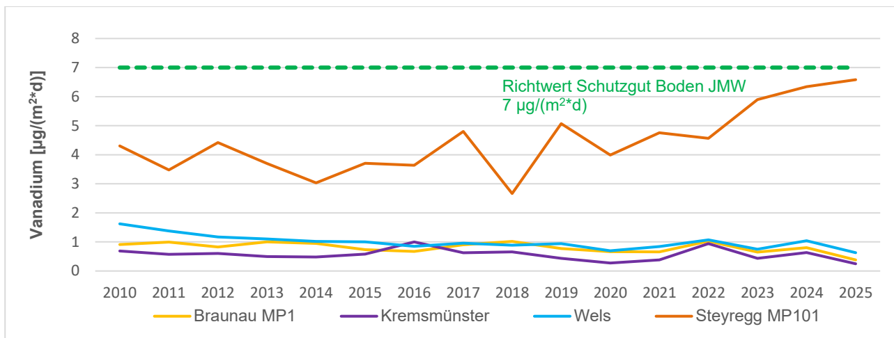
Abbildung 26: Vanadium im JMW im Jahrestrend 2010 – 2025
