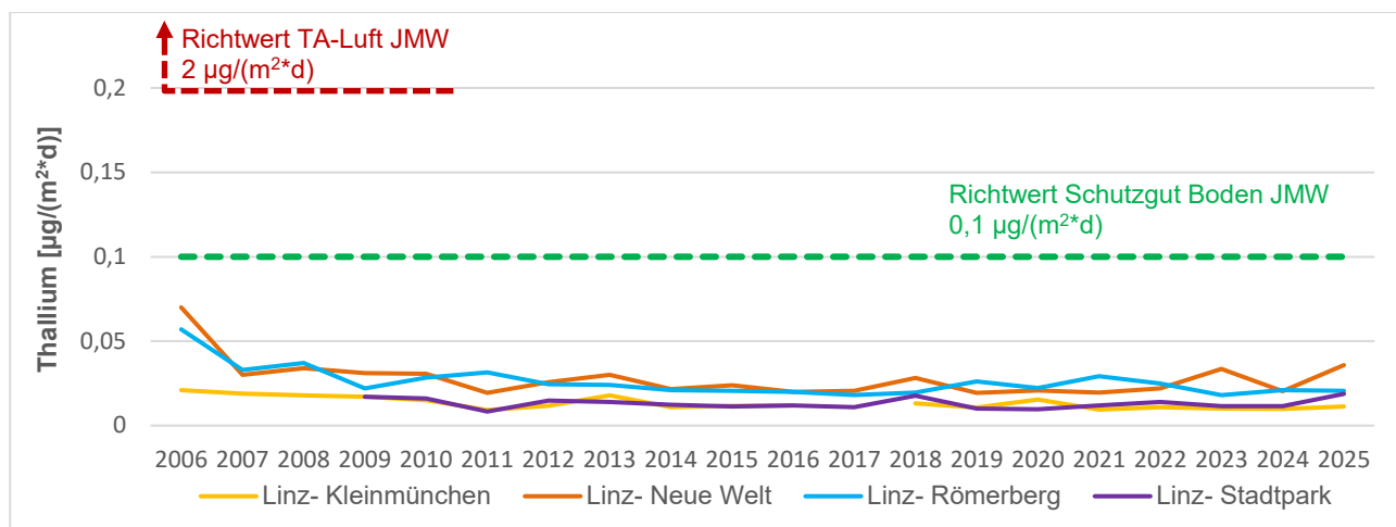
Abbildung 35: Thallium im JMW im Jahrestrend 2006 – 2025
