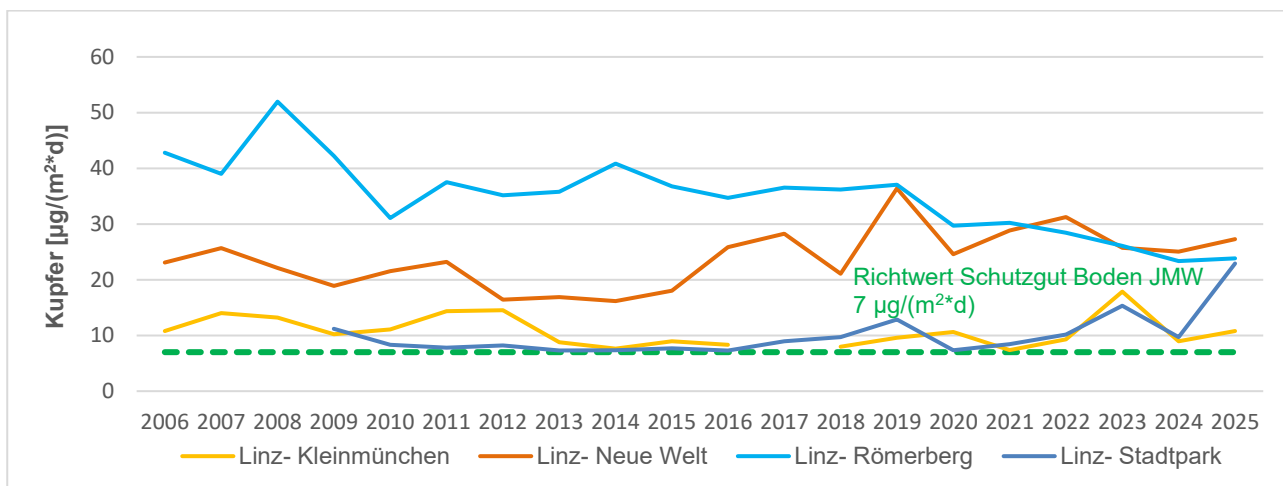
Abbildung 33: Kupfer im JMW im Jahrestrend 2006 – 2025
