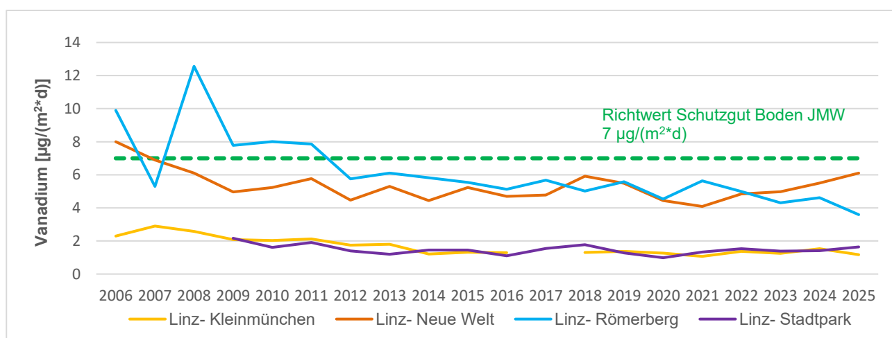
Abbildung 37: Vanadium im JMW im Jahrestrend 2006 – 2025
