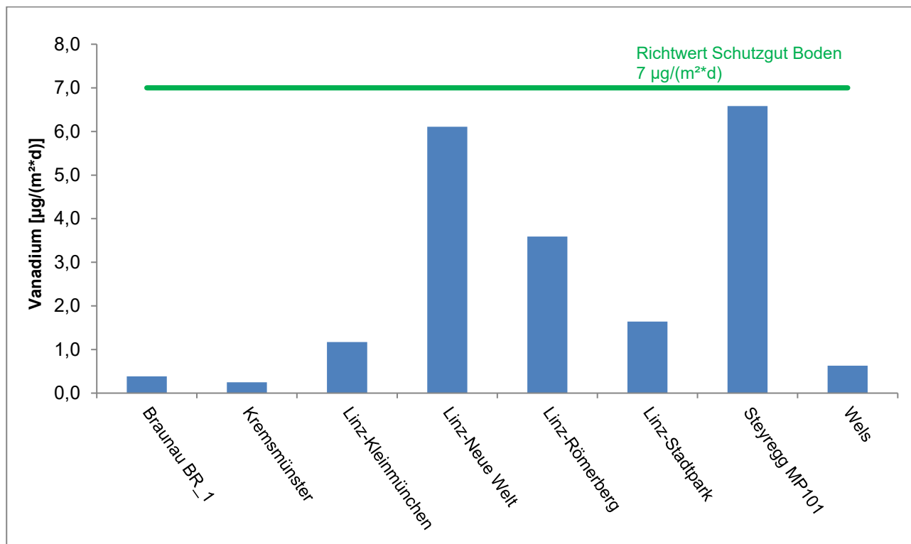
Abbildung 15: Vanadium im JMW der Oö. Messstellen 2025
