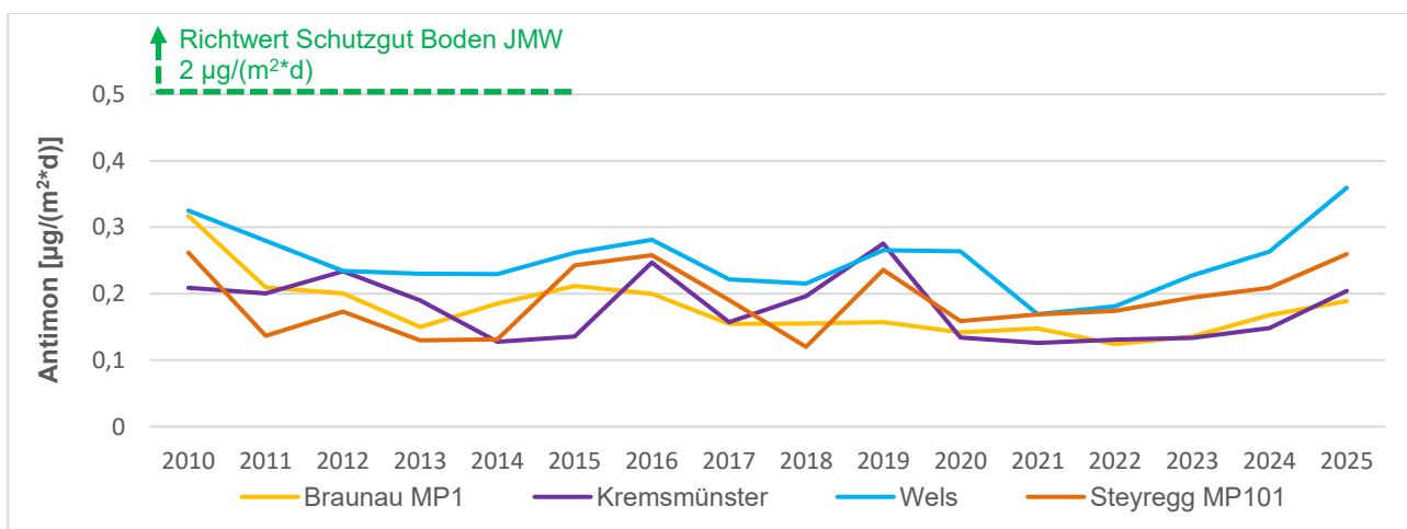
Abbildung 25: Antimon im JMW im Jahrestrend 2010 – 2025
