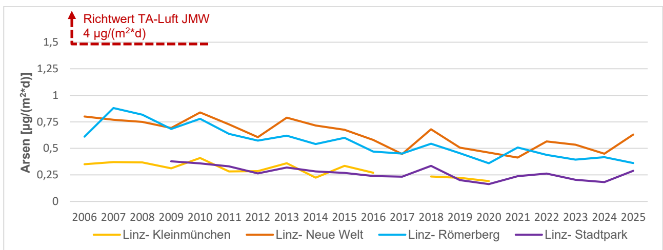
Abbildung 39: Arsen im JMW im Jahrestrend 2006 – 2025
