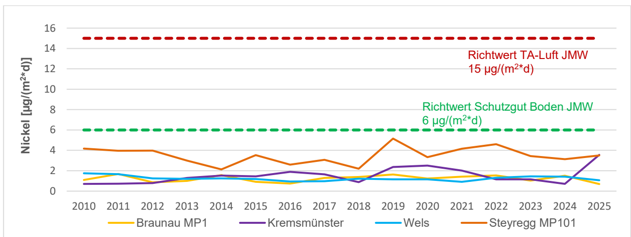
Abbildung 21: Nickel im JMW im Jahrestrend 2010 – 2025
