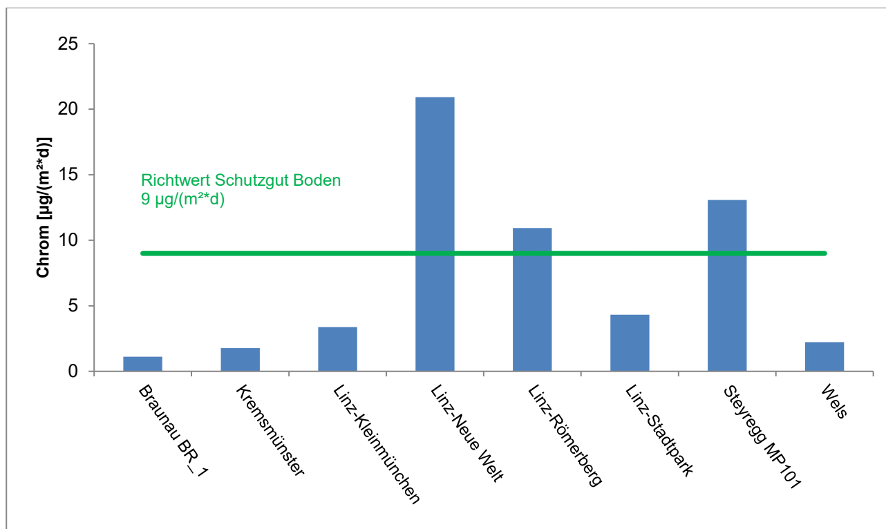
Abbildung 12: Chrom im JMW der Oö. Messstellen 2025
