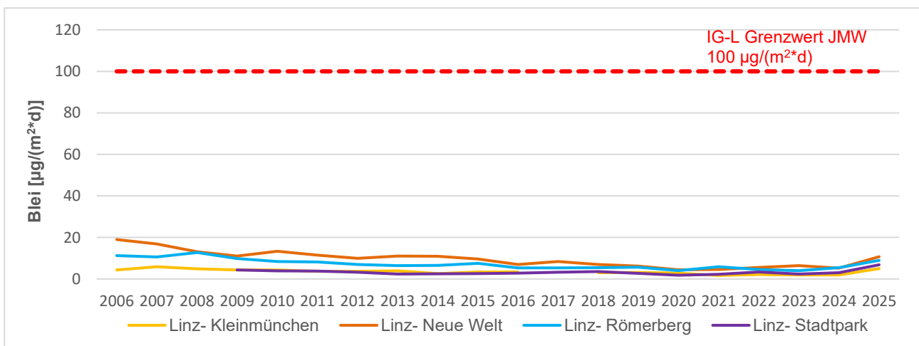
Abbildung 30: Blei im JMW im Jahrestrend 2006 – 2025
