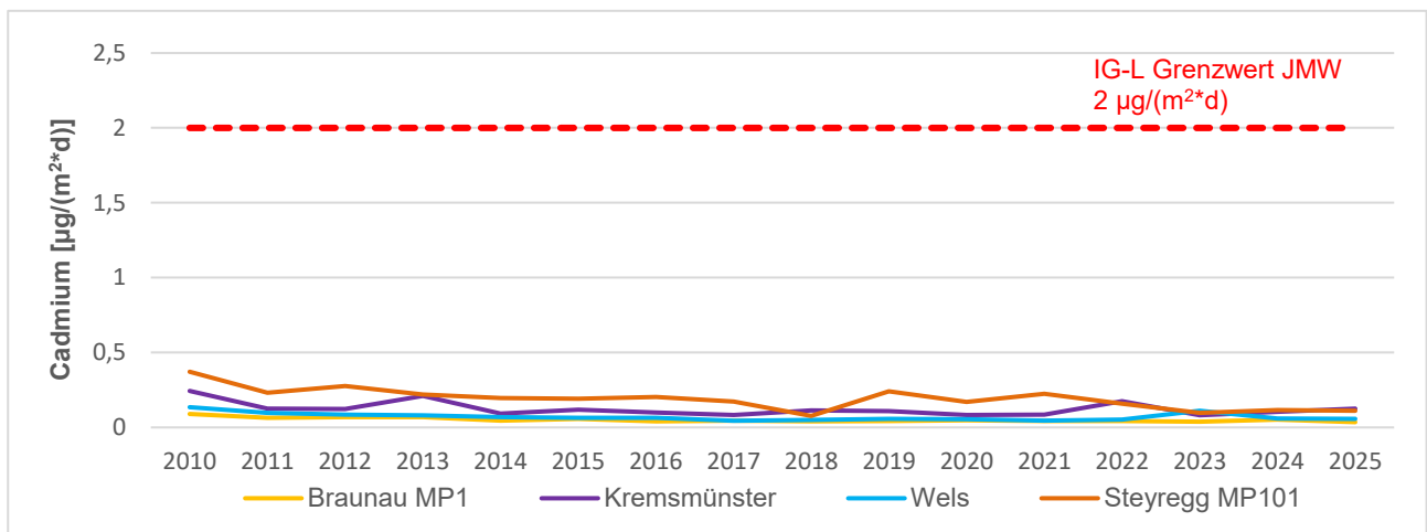
Abbildung 20: Cadmium im JMW im Jahrestrend 2010 – 2025
