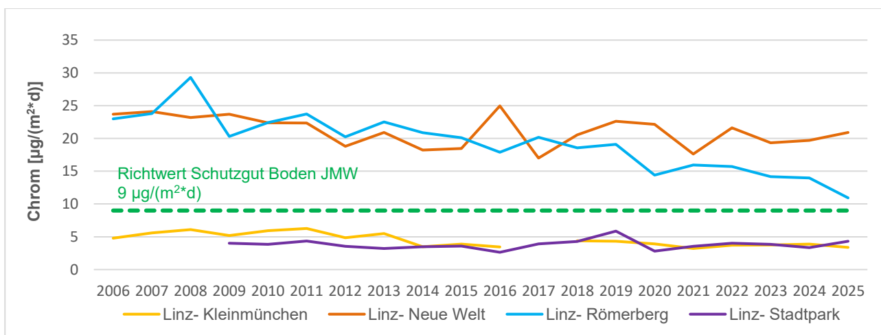
Abbildung 34: Chrom im JMW im Jahrestrend 2006 – 2025
