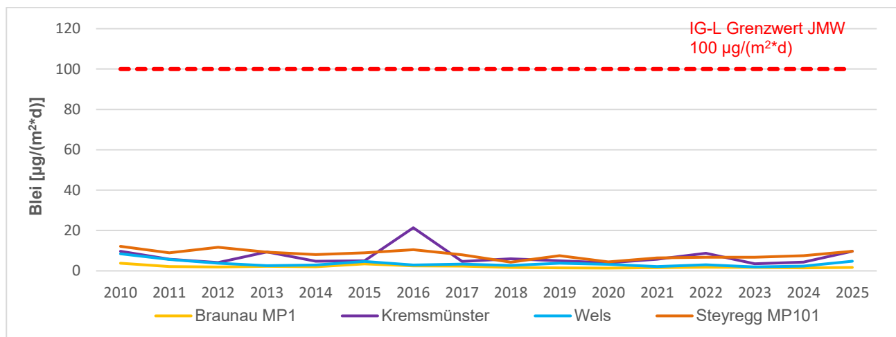
Abbildung 19: Blei im JMW im Jahrestrend 2010 – 2025
