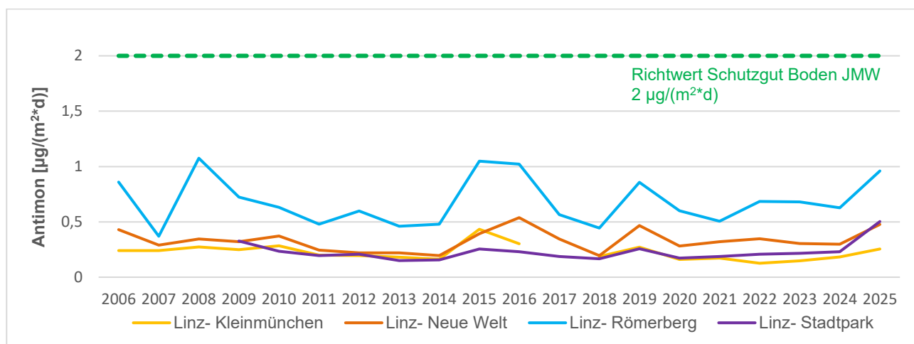
Abbildung 36: Antimon im JMW im Jahrestrend 2006 - 2025
