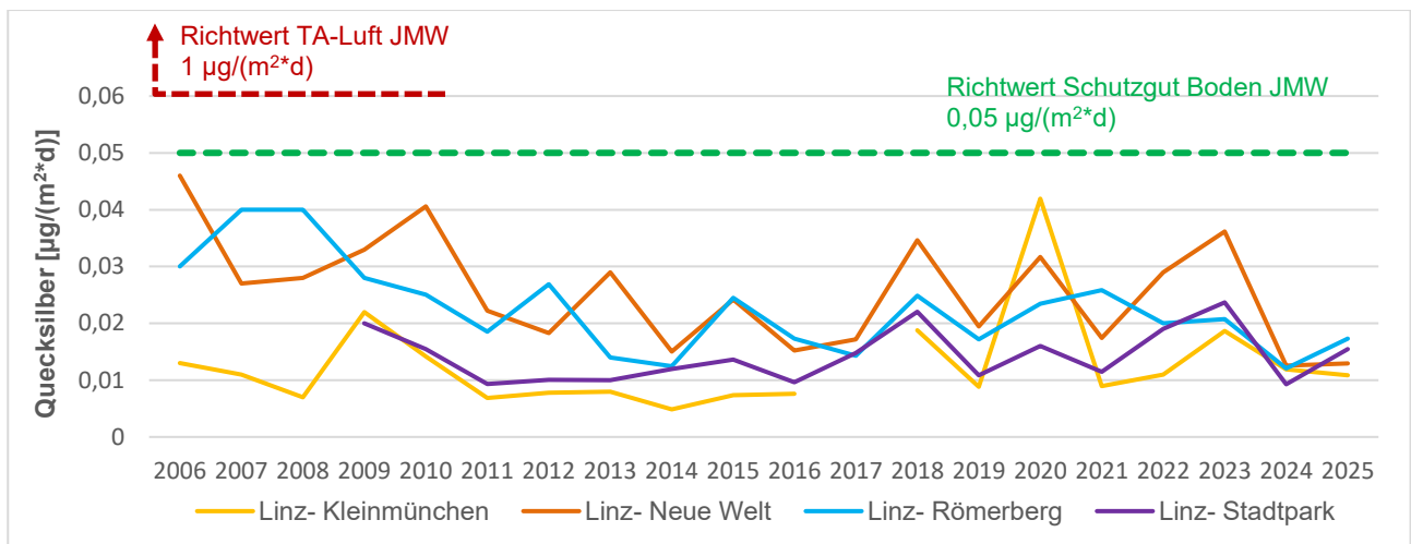
Abbildung 38: Quecksilber im JMW im Jahrestrend 2006 – 2025
