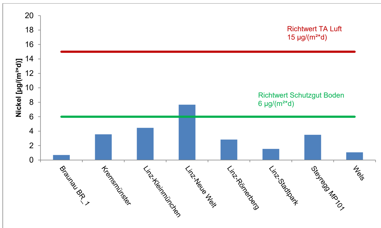
Abbildung 10: Nickel im JMW der Oö. Messstellen 2025
