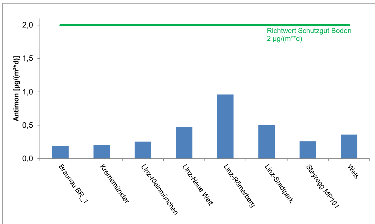
Abbildung 14: Antimon im JMW der Oö. Messstellen 2025
