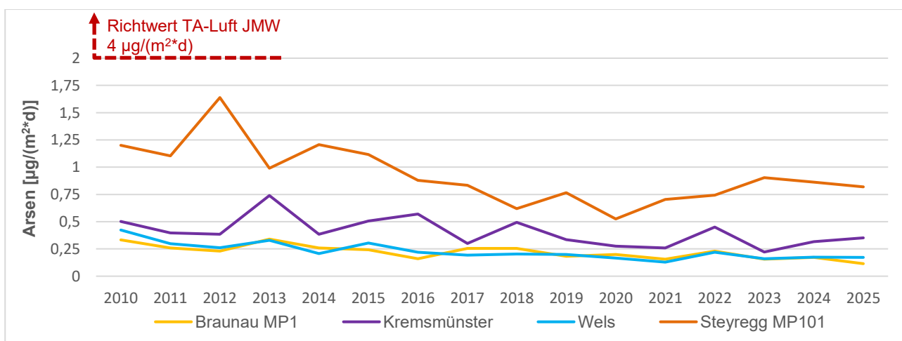
Abbildung 28: Arsen im JMW im Jahrestrend 2010 – 2025
