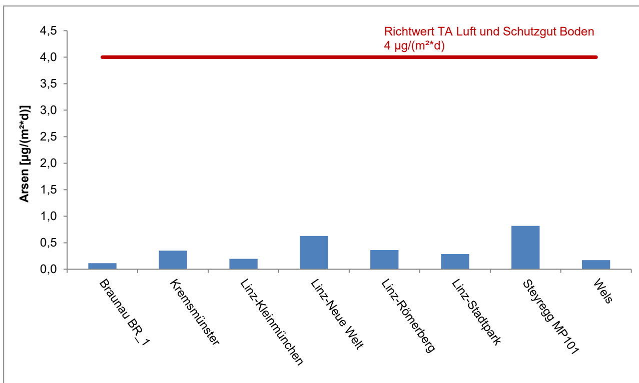
Abbildung 17: Arsen im JMW der Oö. Messstellen 2025
