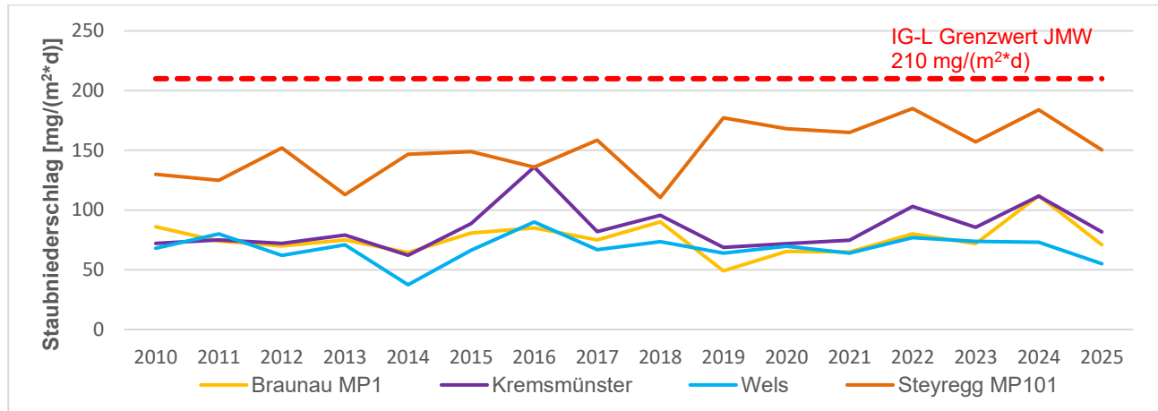
Abbildung 18: Staubniederschlag im JMW im Jahrestrend 2010 – 2025
