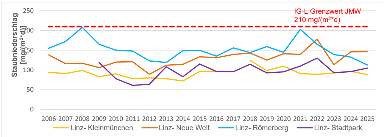
Abbildung 29: Staubniederschlag im JMW im Jahrestrend 2006 – 2025
