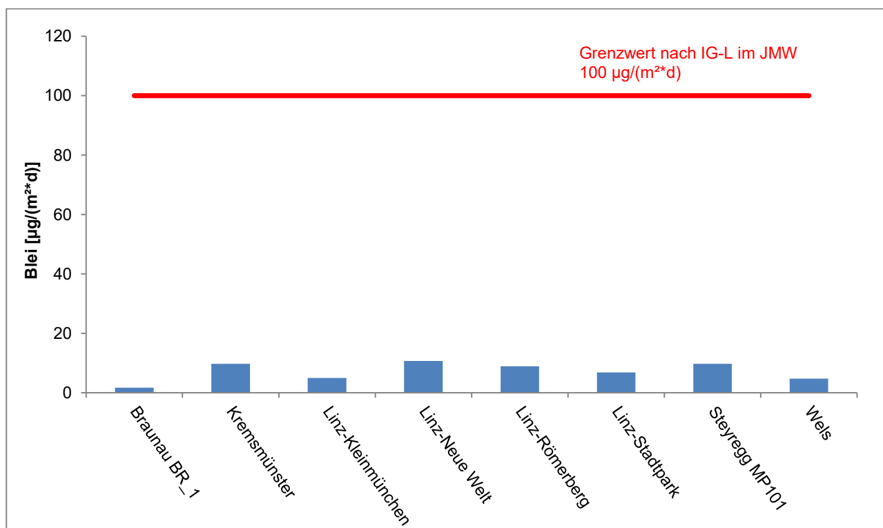
Abbildung 8: Blei im JMW der Oö. Messstellen 2025
