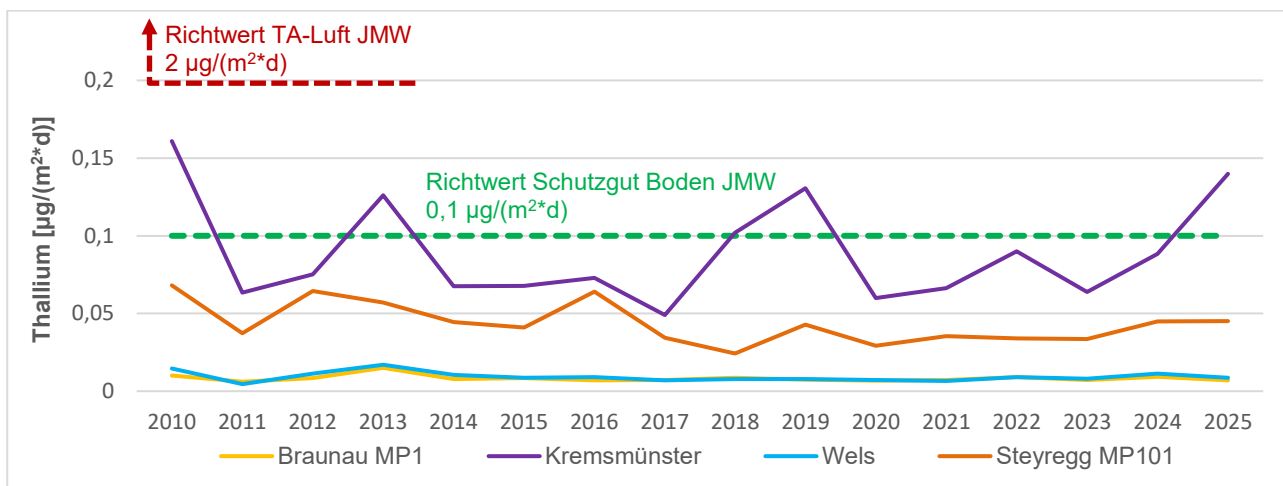
Abbildung 24: Thallium im JMW im Jahrestrend 2010 – 2025
