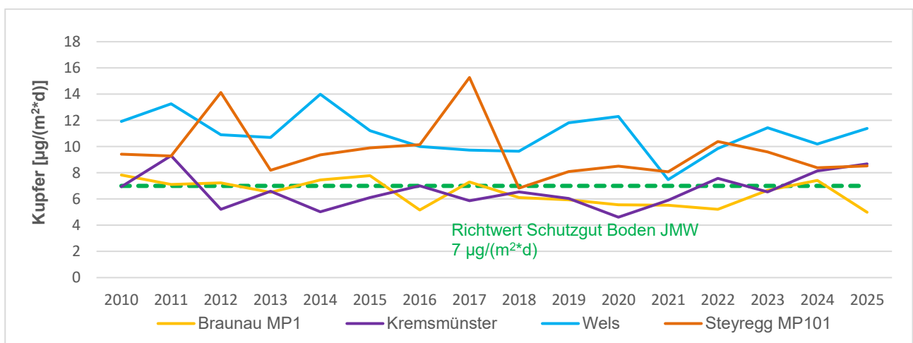
Abbildung 22: Kupfer im JMW im Jahrestrend 2010 – 2025
