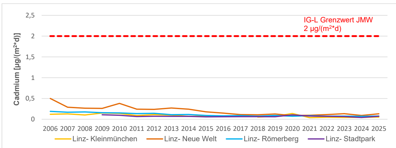
Abbildung 31: Cadmium im JMW im Jahrestrend 2006 – 2025
