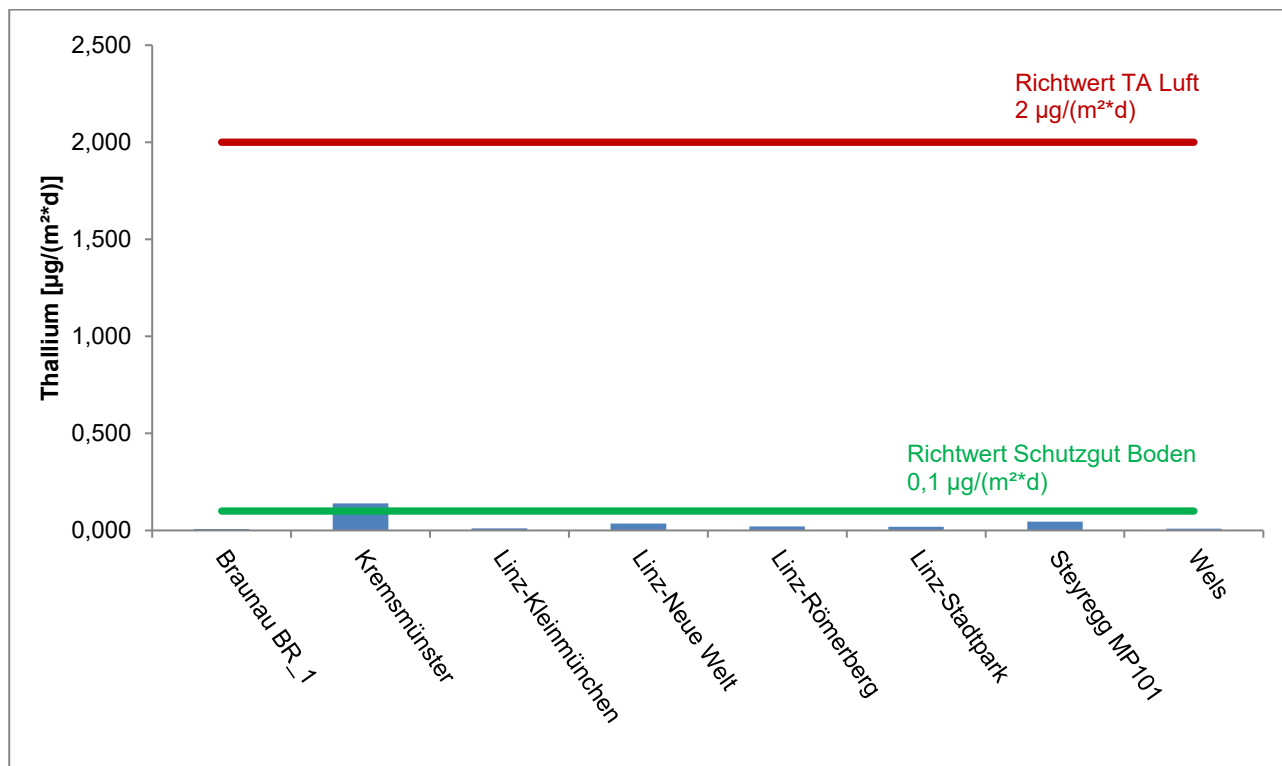
Abbildung 13: Thallium im JMW der Oö. Messstellen 2025
