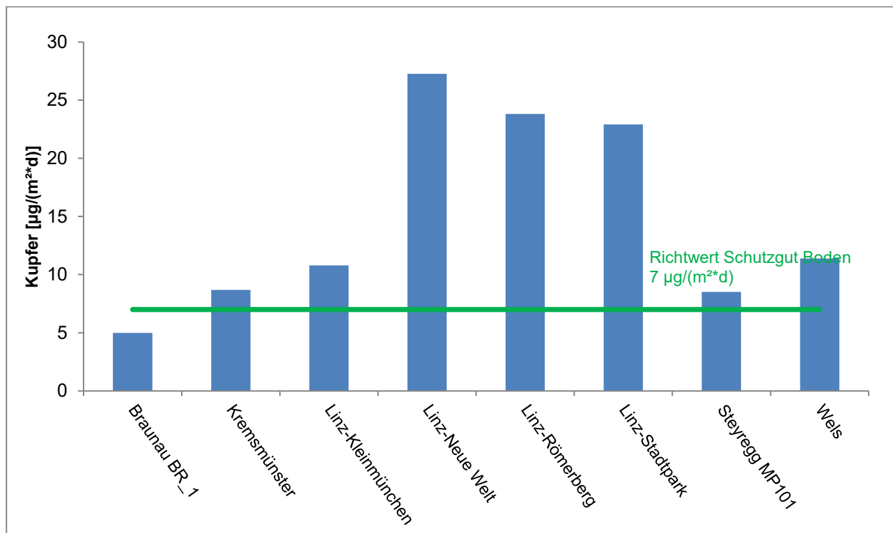
Abbildung 11: Kupfer im JMW der Oö. Messstellen 2025
