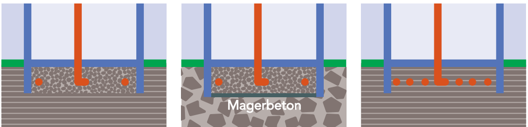
Einbau in Schotter und Kiesbett (Rohrabstand bis zu 8 m)
