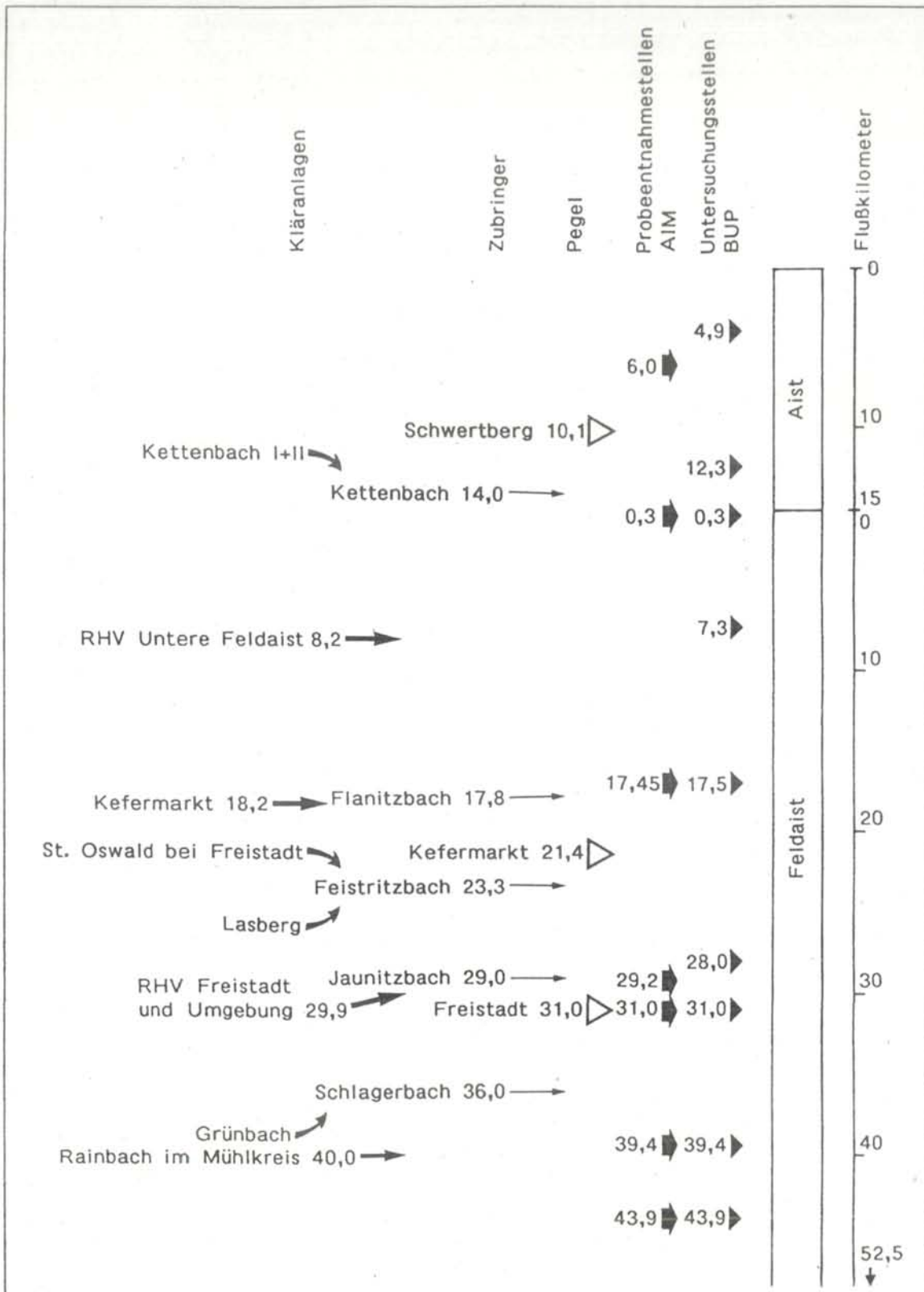
Abb. H5: Längsverlauf der Feldaist und der Aist, schematisch, mit Probeentnahme- und Untersuchungsstellen, Kläranlagen, ausgewählten Zuflüssen und Pegelstellen.
