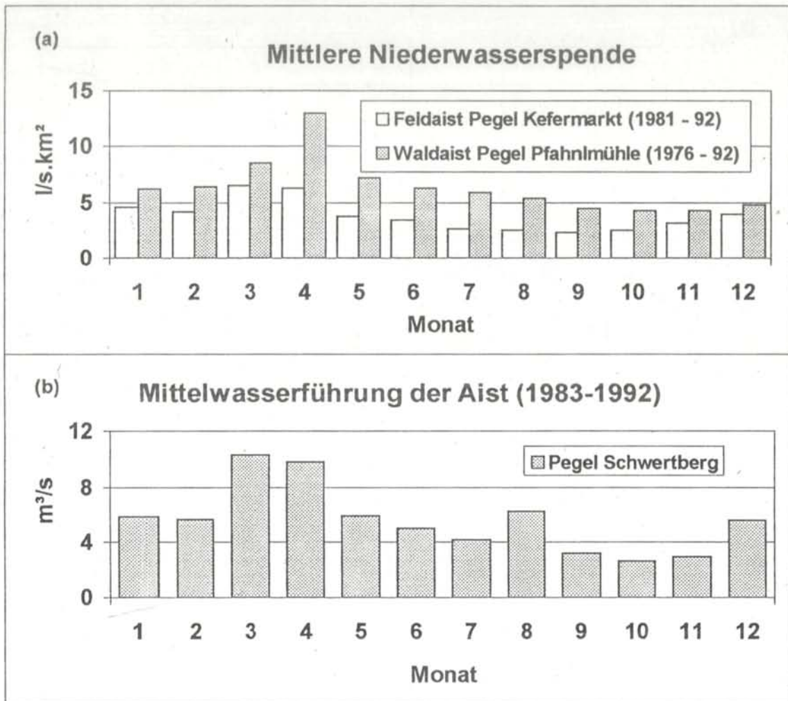
Abb. H3: Abflußverhältnisse im Einzugsgebiet der Aist. (a) Mittlere monatliche Niederwasserspende am Pegel Kefermarkt in der Feldaist (Reihe 1981 bis 1992) und am Pegel Pfahlmühle in der Waldaist (Reihe 1976 bis 1992). (b) Monatsmittel des Abflusses der Aist am Pegel Schwertberg der Reihe 1983 bis 1992. (Daten aus [18]).
