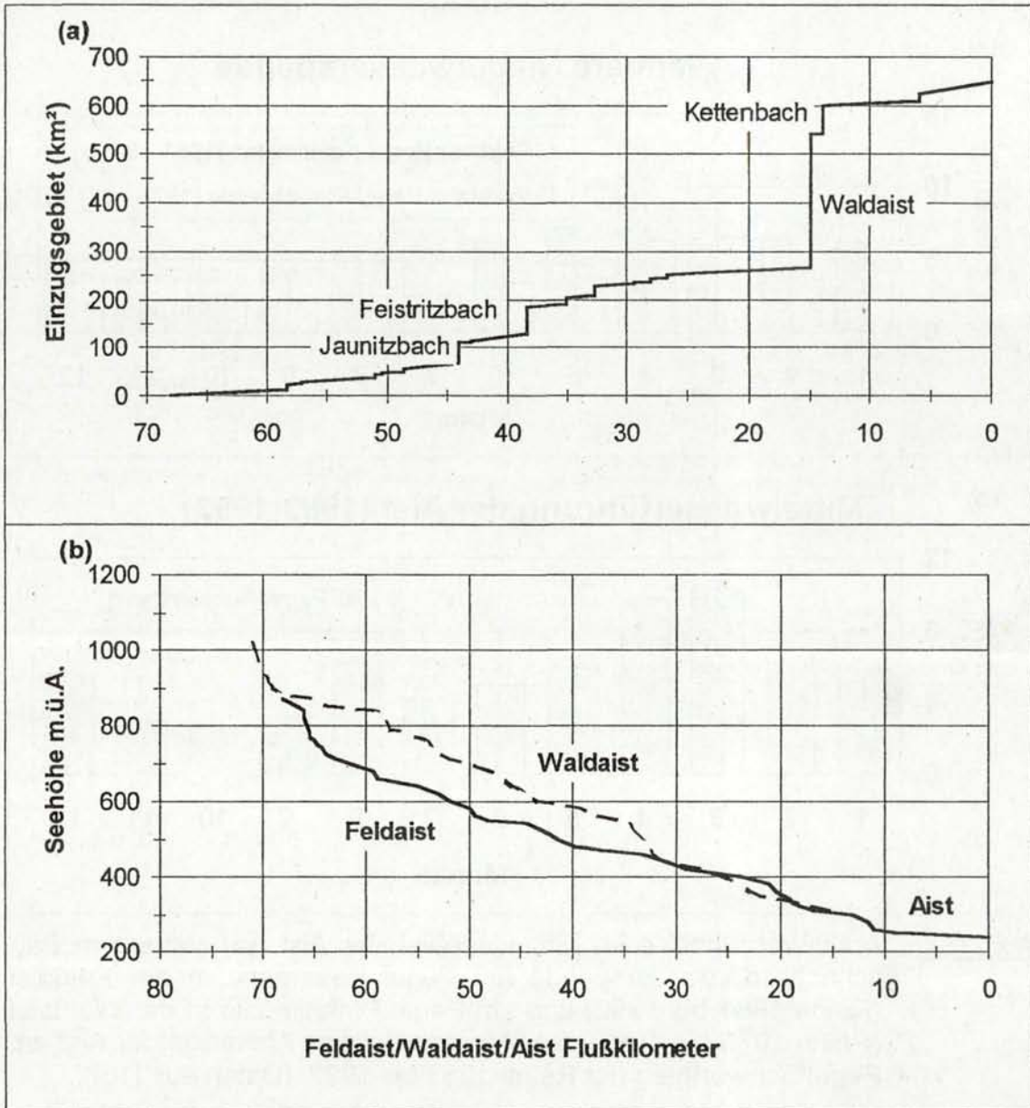
Abb. H2: Schematischer Längsverlauf der Feldaist und der Aist; (a): orografisches Einzugsgebiet mit den wichtigsten Zubringern [19]; (b): Gefällslängsschnitt (Basis: ÖK 1 : 50 000).
