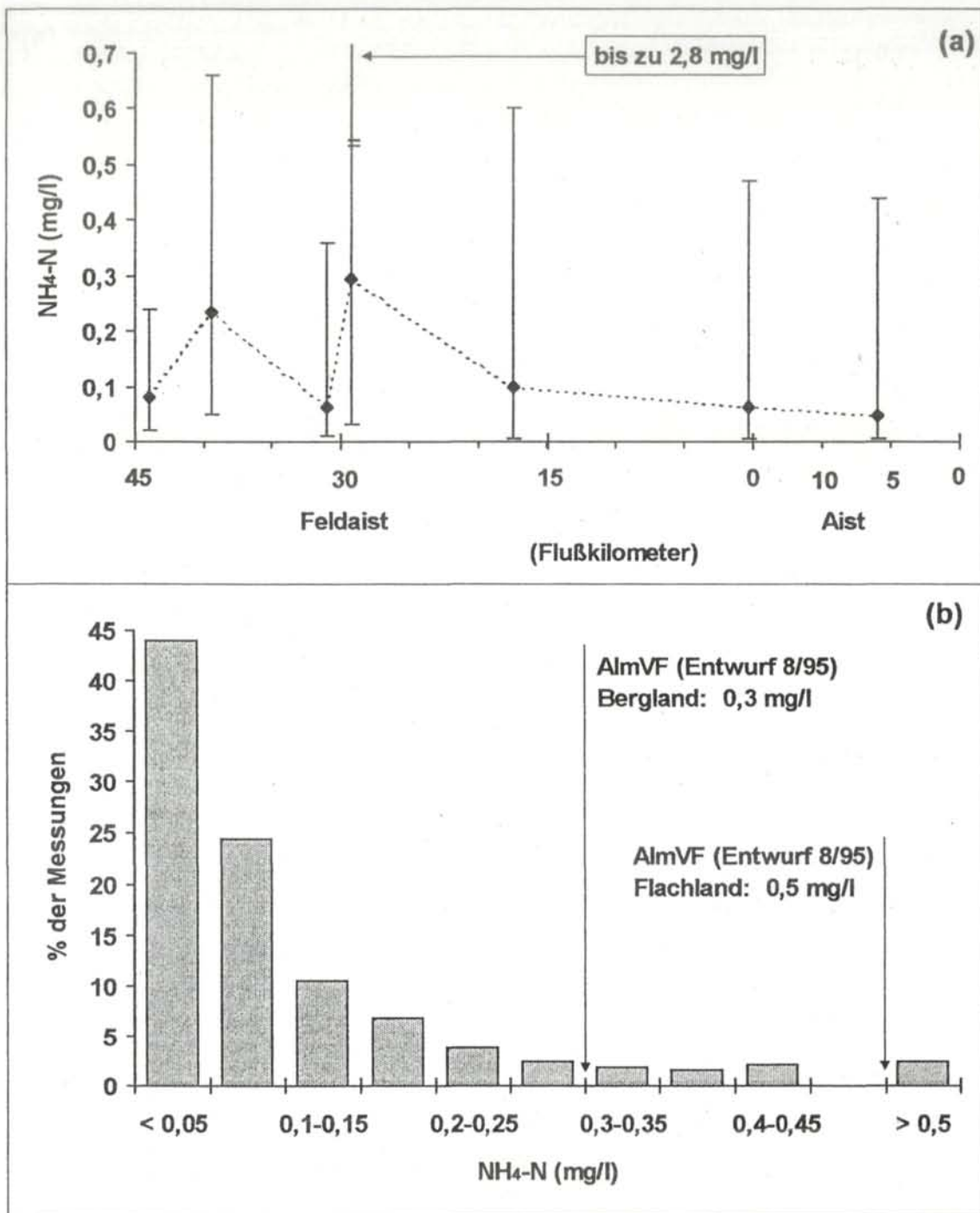
Abb. C5: Ergebnisse der chemisch-physikalischen Untersuchungen der Feldaist und Aist im Beobachtungszeitraum Oktober 1992 bis Mai 1996, Ammonium-Stickstoff. (a): arithmetisches Mittel mit Extremwerten an jeder Probeentnahmestelle, (b): prozentuelle Verteilung aller Werte ( n = 334 ) im Vergleich zu Vorgaben.
