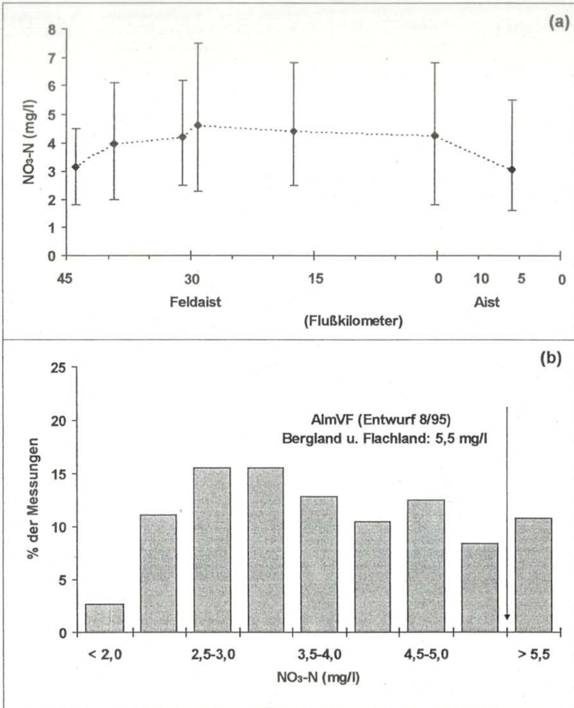
Abb. C7: Ergebnisse der chemisch-physikalischen Untersuchungen der Feldaist und Aist im Beobachtungszeitraum Oktober 1992 bis Mai 1996, Nitrat-N. (a): arithmetisches Mittel mit Extremwerten an jeder Probeentnahmestelle, (b): prozentuelle Verteilung aller Werte (n = 334) im Vergleich zu Vorgaben.
