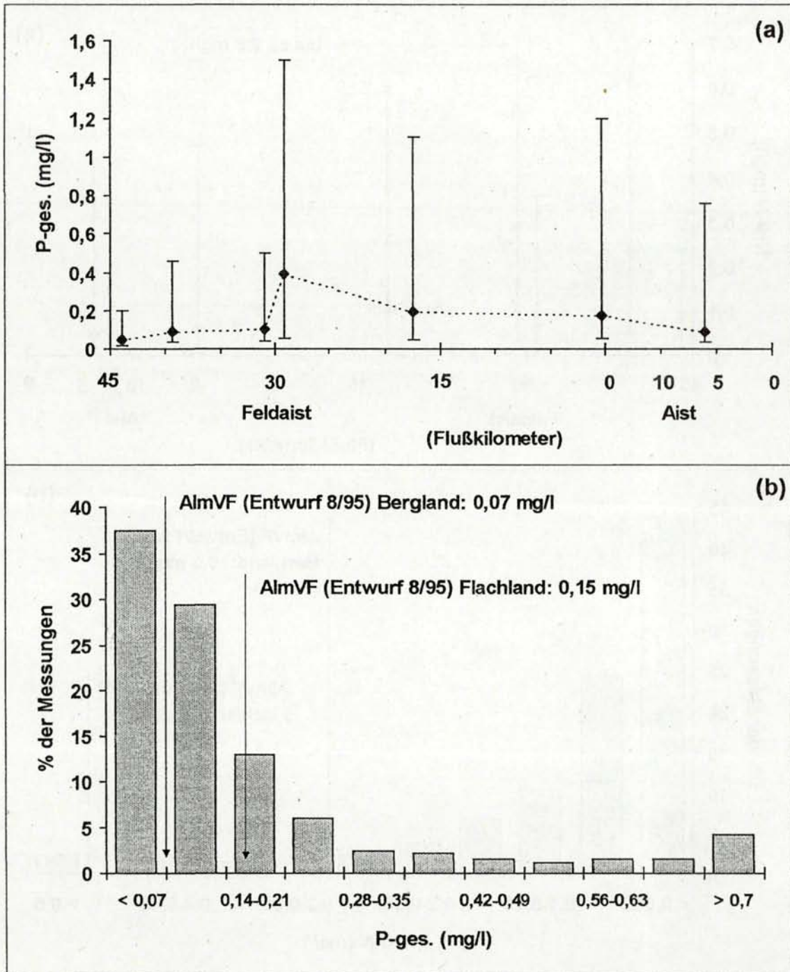
Abb. C4: Ergebnisse der chemisch-physikalischen Untersuchungen der Feldaist und Aist im Beobachtungszeitraum Oktober 1992 bis Mai 1996, Gesamtphosphor. (a): arithmetisches Mittel mit Extremwerten an jeder Probeentnahmestelle, (b): prozentuelle Verteilung aller Werte (n = 334) im Vergleich zu Vorgaben.
