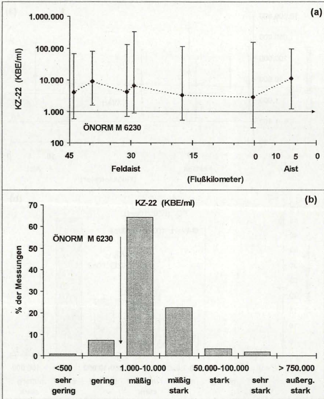
Abb. B1: Ergebnisse der bakteriologischen Untersuchungen der Feldaist und Aist im Beobachtungszeitraum Oktober 1992 bis Mai 1996, KZ-22, (a): geometrisches Mittel mit Extremwerten an jeder Probenentnahmestelle, (b): prozentuelle Verteilung aller Werte (n = 334) im Vergleich zu Vorgaben.
