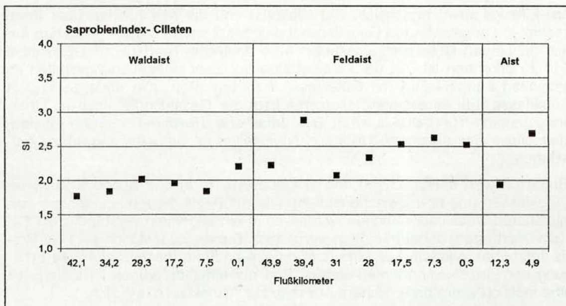
Abb. C12: Ciliaten, errechneter Saprobienindex im Längsverlauf der Waldaist, Feldaist und Aist.
