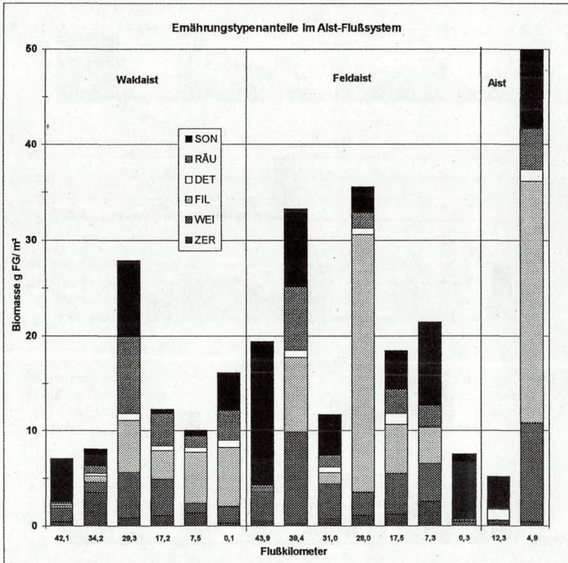
Abb. M1: Makrozoobenthos, Abundanz (Biomasse-Formolfrischgewicht \text{g/m}^2 ) der Ernährungstypen im Längsverlauf der Waldaist, Feldaist und Aist. Taxonomische Gruppen, die mehrere Typen repräsentieren, wurden dem Typ zugeordnet, der dem überwiegenden Anteil entspricht; ZER = Zerkleinerer, WIE = Weidegänger, FIL = Filtrierer, DET = Detritivore, RÄU = Räuber, SON = Sonstige.
