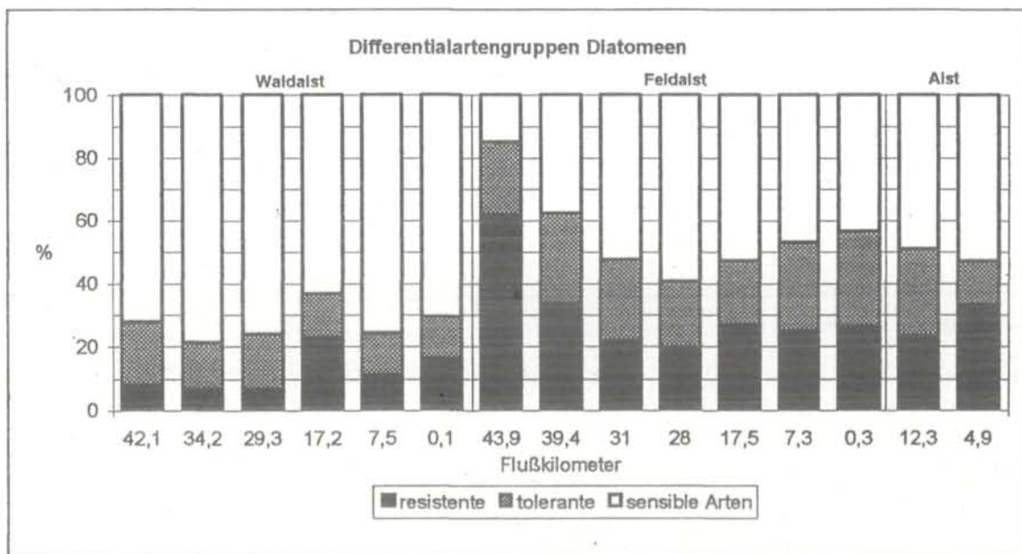
Abb. D1: Diatomeen, relative Häufigkeit der Differentialartengruppen in der Waldaist, Feldaist und Aist.
