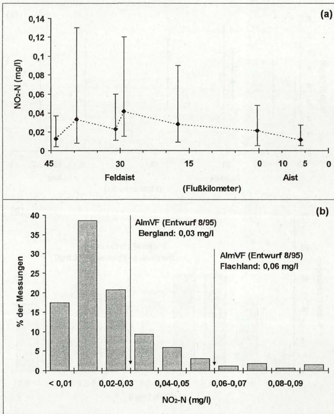
Abb. C6: Ergebnisse der chemisch-physikalischen Untersuchungen der Feldaist und Aist im Beobachtungszeitraum Oktober 1992 bis Mai 1996, Nitrit-N. (a): arithmetisches Mittel mit Extremwerten an jeder Probeentnahmestelle, (b): prozentuelle Verteilung aller Werte (n = 334) im Vergleich zu Vorgaben.
