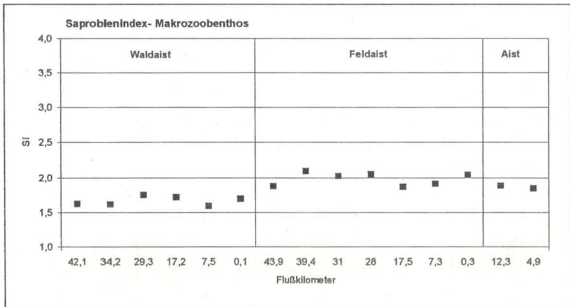
Abb. M 4: Makrozoobenthos, errechneter Saprobienindex im Längsverlauf der Waldaist, Feldaist und Aist.
