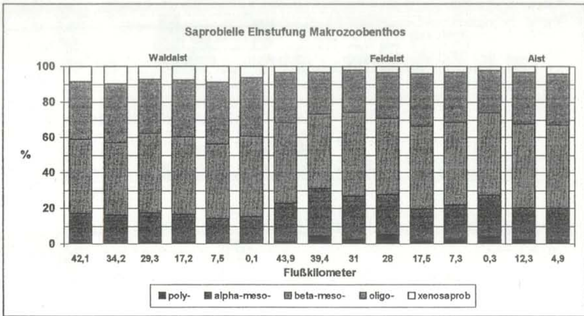
Abb. M3: Makrozoobenthos, saprobielle Einstufung im Längsverlauf der Waldaist, Feldaist und Aist; relative Häufigkeit in den saprobiellen Stufen.
