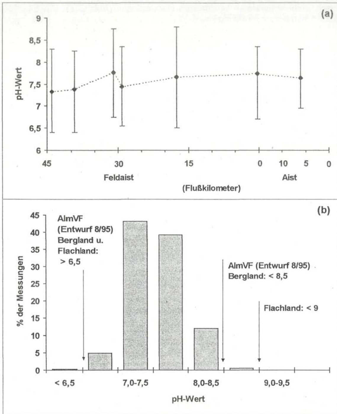
Abb. C1: Ergebnisse der chemisch-physikalischen Untersuchungen der Feldaist und Aist im Beobachtungszeitraum Oktober 1992 bis Mai 1996, pH-Wert. (a): arithmetisches Mittel mit Extremwerten an jeder Probeentnahmestelle, (b): prozentuelle Verteilung aller Werte (n = 334) im Vergleich zu Vorgaben.
