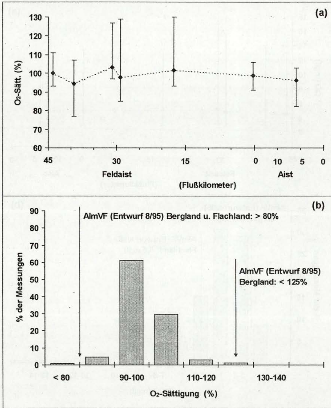
Abb. C2: Ergebnisse der chemisch-physikalischen Untersuchungen der Feldaist und Aist im Beobachtungszeitraum Oktober 1992 bis Mai 1996, Sauerstoff-Sättigung (%). (a): arithmetisches Mittel mit Extremwerten an jeder Probeentnahmestelle, (b): prozentuelle Verteilung aller Werte (n = 334) im Vergleich zu Vorgaben.
