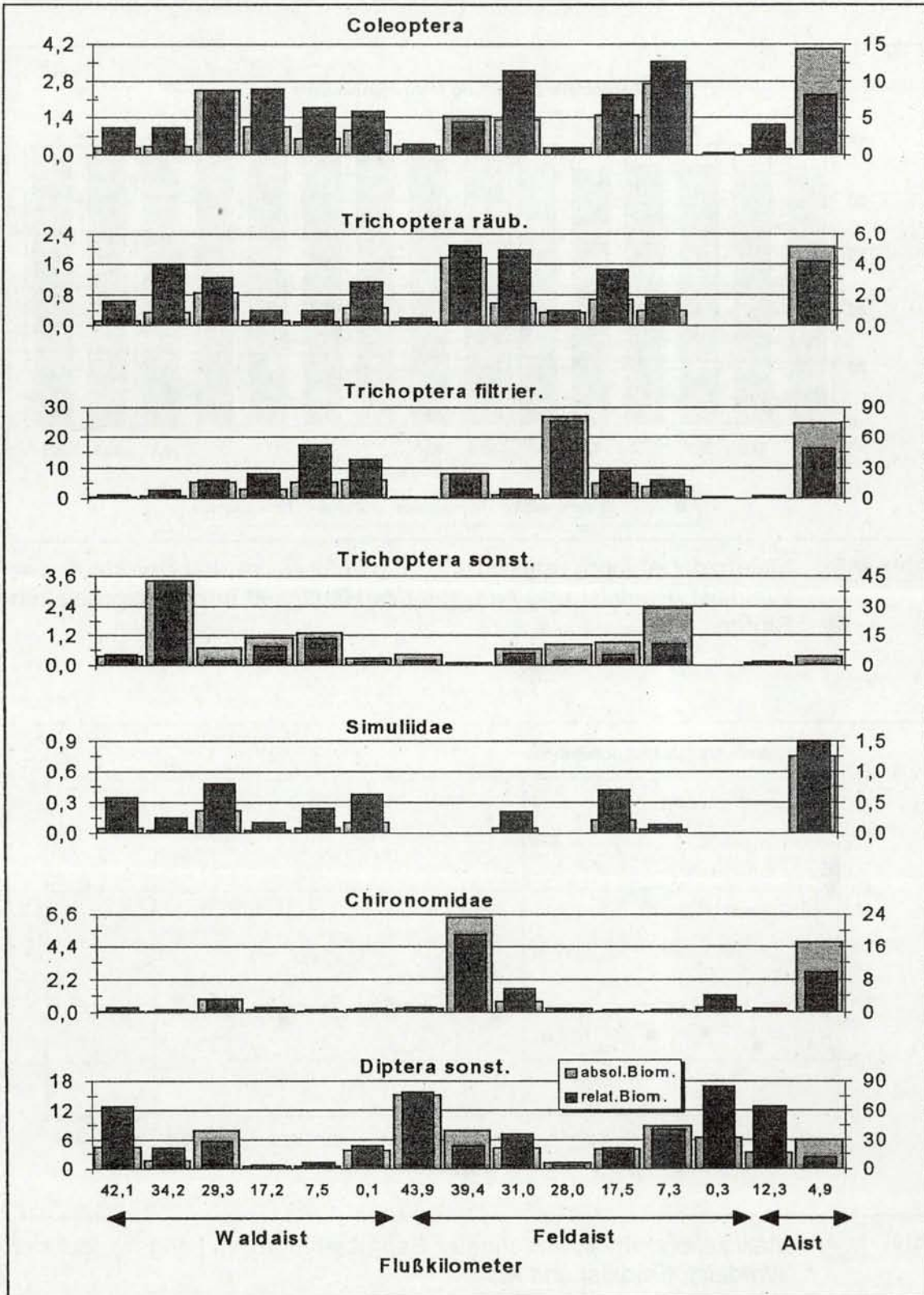
Abb. M2: Makrozoobenthos, absolute (Biomasse, Formolfrischgewicht g/m 2 ) und relative Abundanz der taxonomischen Gruppen im Längsverlauf der Waldaist, Feldaist und Aist; y-Achse rechts: %, y-Achse links: FG g/m 2 .
