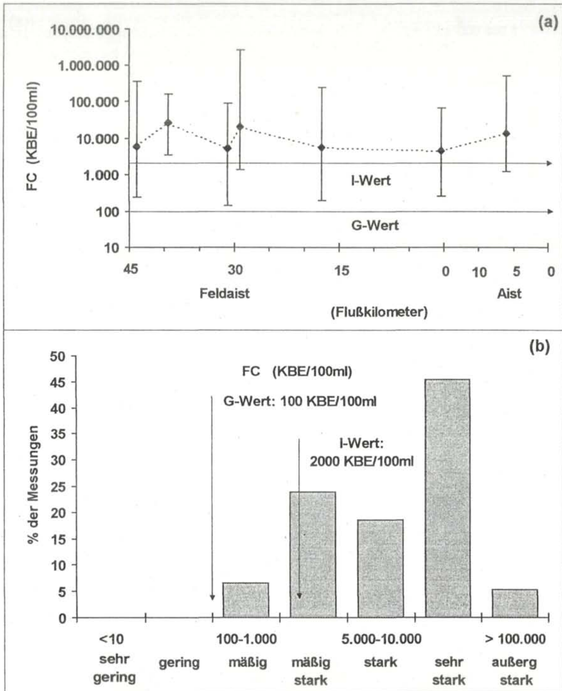
Abb. B2: Ergebnisse der bakteriologischen Untersuchungen der Feldaist und Aist im Beobachtungszeitraum Oktober 1992 bis Mai 1996, FC, (a): geometrisches Mittel mit Extremwerten an jeder Probenentnahmestelle, (b): prozentuelle Verteilung aller Werte (n = 334) im Vergleich zu Vorgaben.
