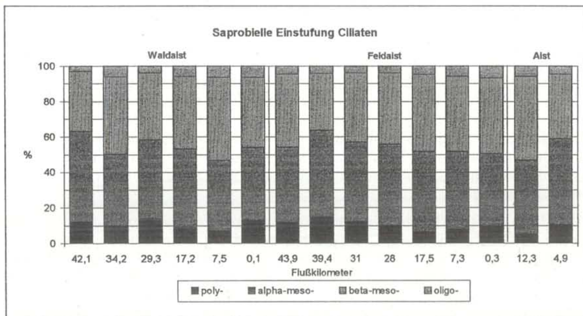
Abb. C11: Ciliaten, saprobielle Einstufung im Längsverlauf der Waldaist, Feldaist und Aist; relative Häufigkeit in den saprobiellen Stufen.
