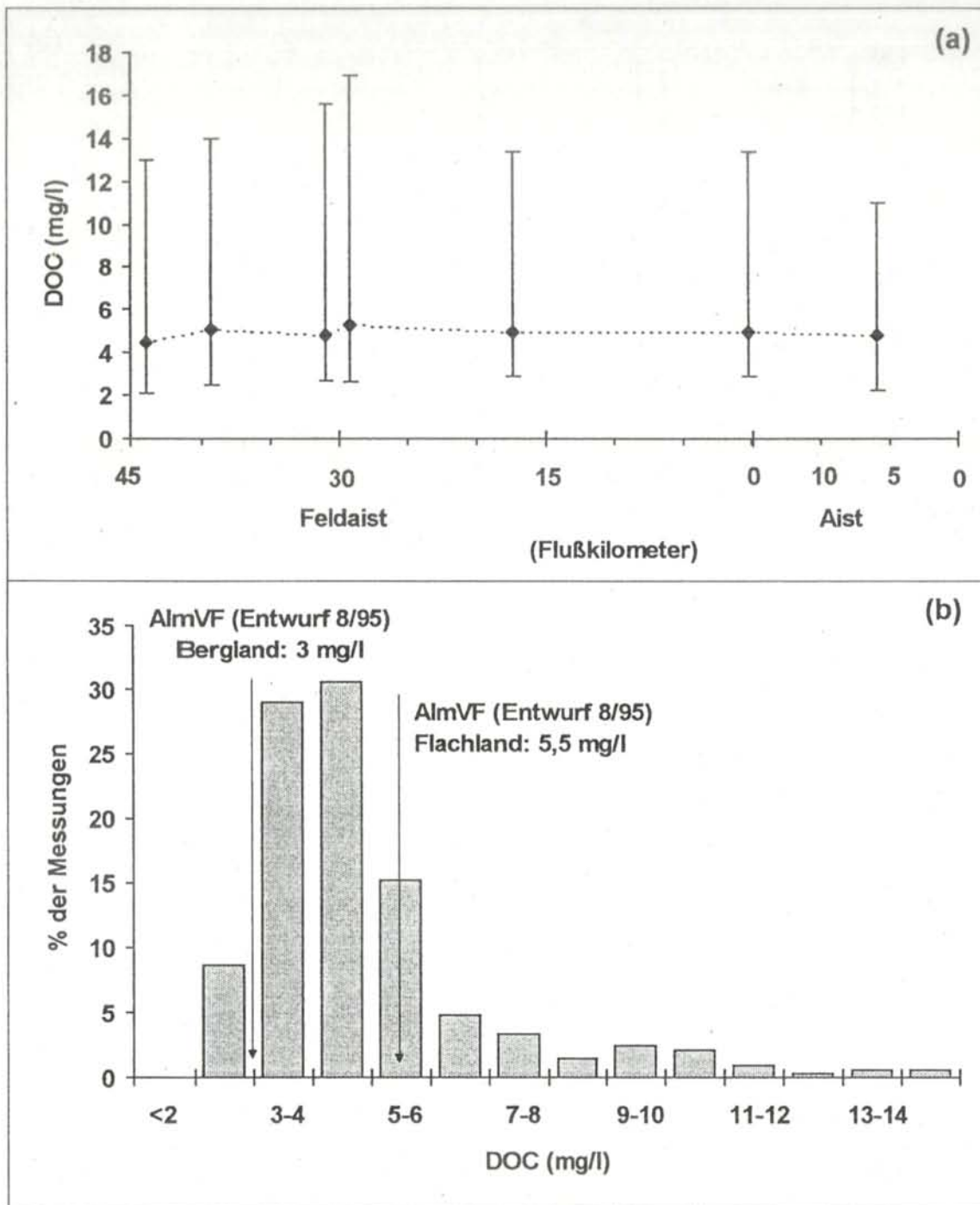
Abb. C3: Ergebnisse der chemisch-physikalischen Untersuchungen der Feldaist und Aist im Beobachtungszeitraum Oktober 1992 bis Mai 1996, DOC. (a): arithmetisches Mittel mit Extremwerten an jeder Probeentnahmestelle, (b): prozentuelle Verteilung aller Werte (n = 334) im Vergleich zu Vorgaben.
