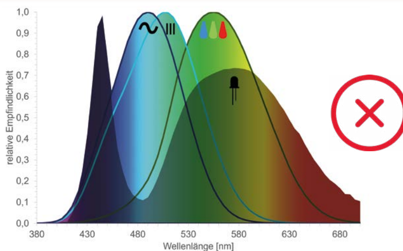
Abb. 21: Spektrum einer neutralweißen LED, im Hintergrund: Empfindlichkeiten der circadianen Rezeptoren für die Steuerung des Tag-Nacht-Rhythmus (links), der Stäbchen (Nachtsehen, Mitte) und der Zapfen (Tagsehen, rechts)
