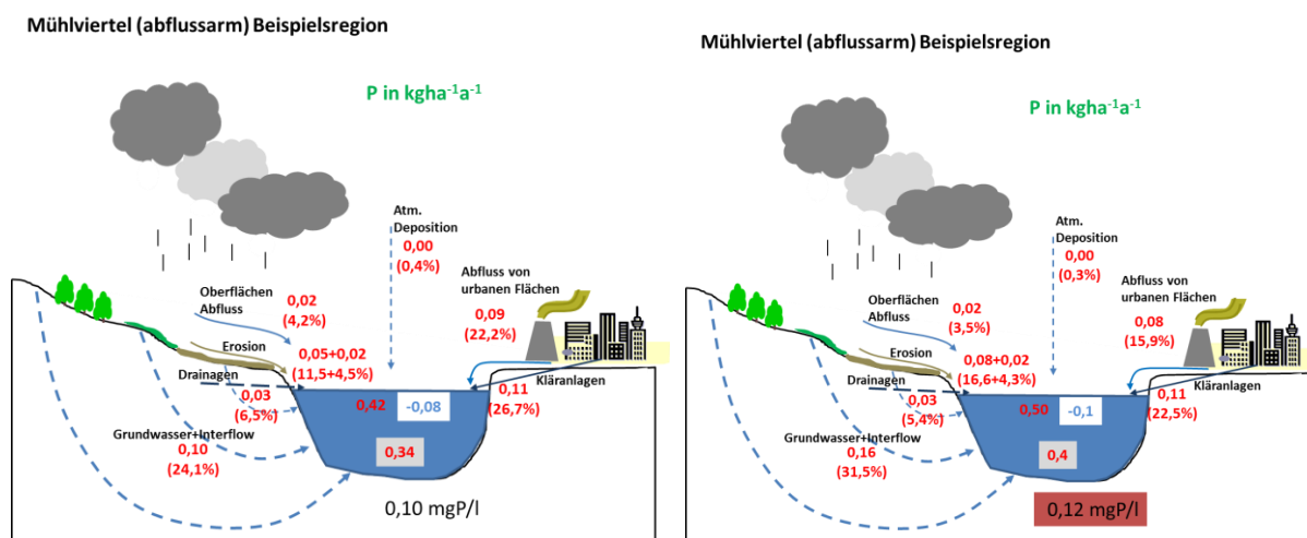
Abbildung 14: P Einträge, Retention und transportierte Fracht [ \text{kg P/ha} \cdot \text{a} ] sowie resultierende mittlere Konzentrationen der Gewässer der Beispielsregion Mühlviertel (abflussarm bzw. Ost) für Projekt „Stoffströme“ (links) im Vergleich zu Projekt „Maßnahmenwirkung“ (rechts)
