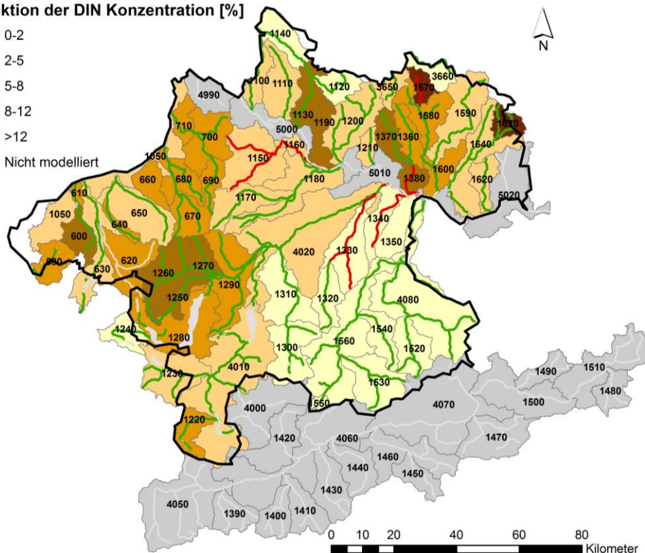
Abbildung 29: Räumliche Darstellung der modellierten Reduktion von DIN-Konzentrationen durch flächendeckende Einführung der Maßnahme „Düngebeschränkung mittlere Ertragslage“. Die in Abbildung 28 bereits berücksichtigten Reduktionen sind nicht dargestellt. Zudem sind Gewässer mit durch Messungen ausgewiesenen Überschreitungen des UQZ dargestellt
