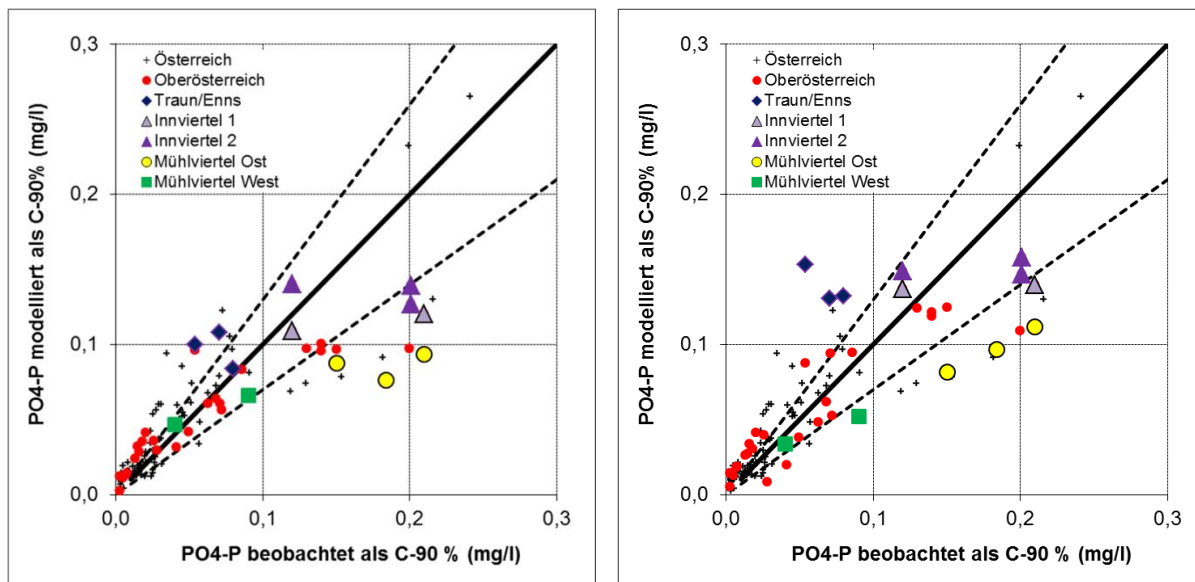
Abbildung 5: Beobachtete und im Projekt „Nährstoffströme“ (links) bzw. im Projekt „Maßnahmenwirkung“ (rechts) modellierte 90% Perzentile der \text{PO}_4\text{-P} Konzentrationen am Gebietsauslass der Modelleinzugsgebiete im Zeitraum 2001-2006
