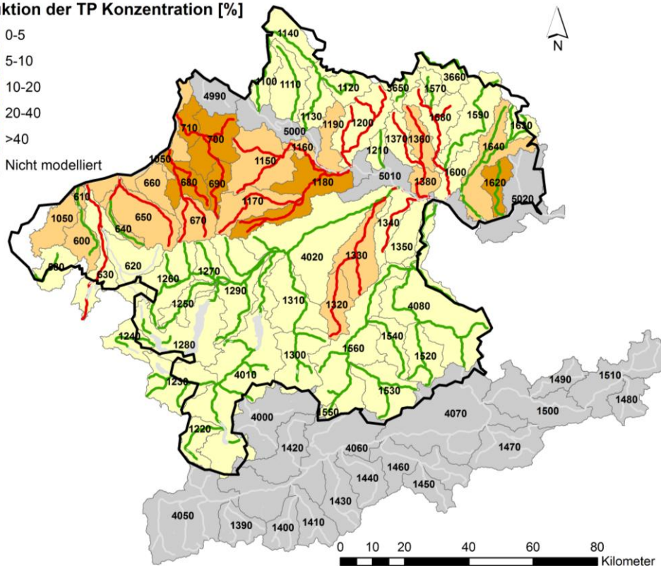
Abbildung 24: Räumliche Darstellung der modellierten Reduktion von TP-Konzentrationen durch flächendeckende Einführung der Maßnahme „Fruchtfolgeauflagen auf steilen Hängen“. Zudem sind Gewässer mit durch Messungen ausgewiesenen Überschreitungen des UQZ dargestellt
