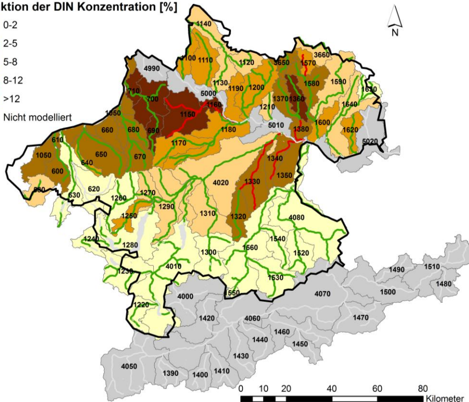
Abbildung 30: Räumliche Darstellung der modellierten Reduktion von DIN-Konzentrationen durch flächendeckende Einführung der Maßnahme „Düngung nach Bodenvorrat“. Die in Abbildung 28 bereits berücksichtigten Reduktionen sind nicht dargestellt. Zudem sind Gewässer mit durch Messungen ausgewiesenen Überschreitungen des UQZ dargestellt
