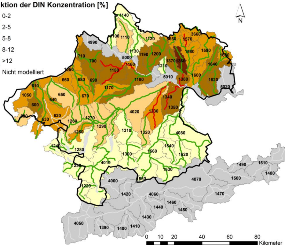
Abbildung 28: Räumliche Darstellung der modellierten Reduktion von DIN-Konzentrationen in den Fließgewässern, welche aufgrund bereits umgesetzter Maßnahmen noch zu erwarten sind. Zudem sind Gewässer mit durch Messungen ausgewiesenen Überschreitungen des UQZ dargestellt
