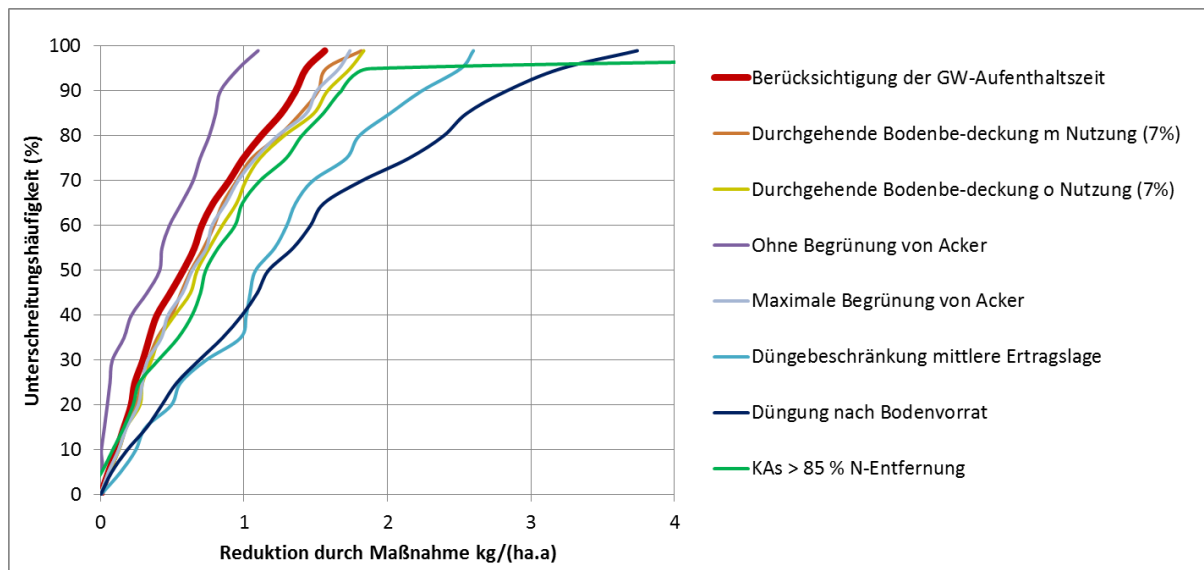
Abbildung 26: Unterschreitungshäufigkeit der TN-Emissionsreduktion durch unterschiedliche Maßnahmen auf Ebene von Teileinzugsgebieten. Die Auswirkungen der Maßnahmen sind additive zu den Auswirkungen, welche sich lediglich durch Berücksichtigung der Grundwasseraufenthaltszeit ergeben, dargestellt
