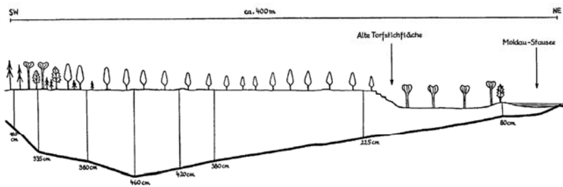
Abb. 28: Bohr-Längsprofil durch die Bayerische Au (DUNZENDORFER 1974)
