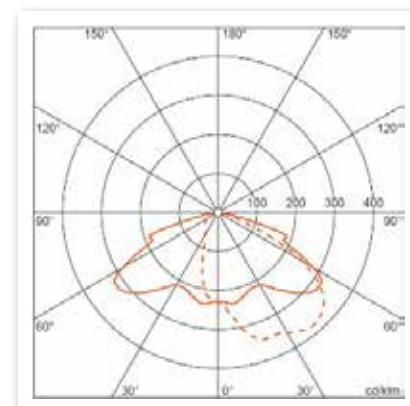
typische Lichtverteilung Full-Cut-Off Leuchte
