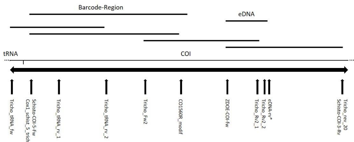
Abb. 4: Positionen der verwendeten PCR-Primer für die COI -Sequenz auf Basis der COI -Sequenz von Trichobilharzia szidati (NCBI: MG570047.1). Die Pfeile markieren die Position der entwickelten Primer (ein Primer-Paar flankiert dabei jeweils das amplifizierte Fragment). Die beiden obersten Linien entsprechen der Barcode-Region (Folmer-Region) sowie dem verwendeten eDNA-Abschnitt. Die vier anderen Linien repräsentieren die im Projekt am häufigsten generierten Teil-Fragmente.
