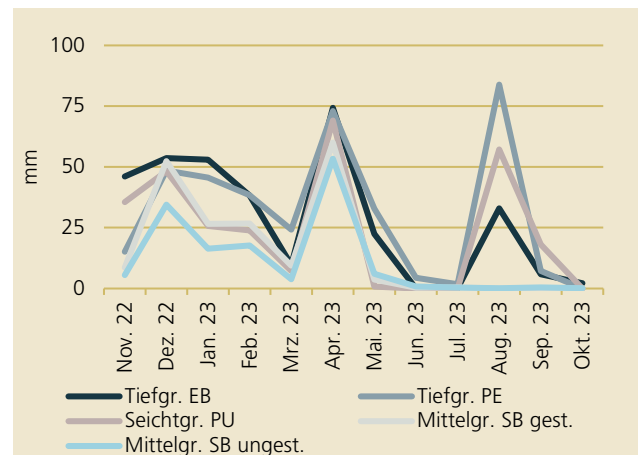
Abb. 5-32: Monatliche Sickerwassermengen
