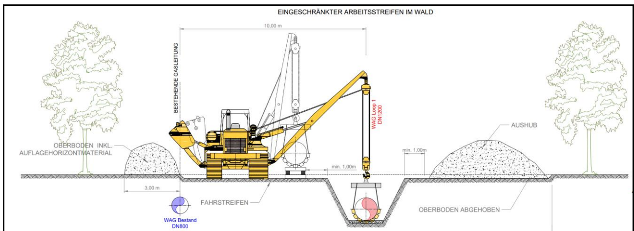
Screenshot – Technisches Projekt (B.01.104) – Skizze Regelprofil Wald
