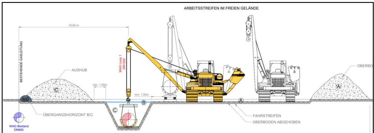
Screenshot – Technisches Projekt (B.01.104) – Skizze Regelprofil freies Gelände
