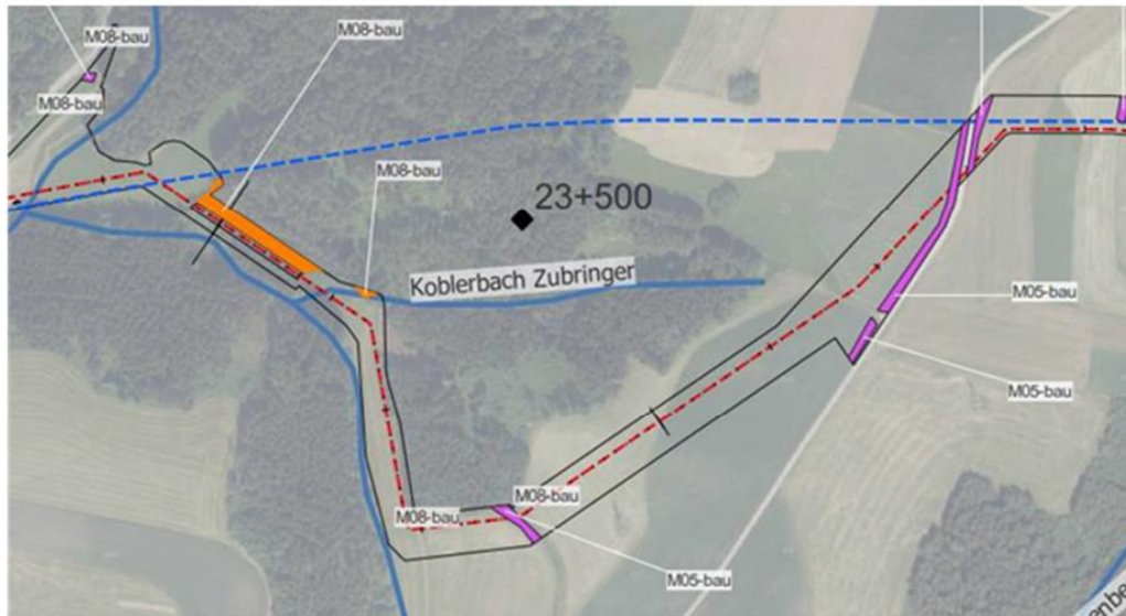
Abbildung: Abweichung im Bereich zwischen den Leitungskilometer km 23+160 bis km 24+070; Quelle Maßnahmenplan Rev A
