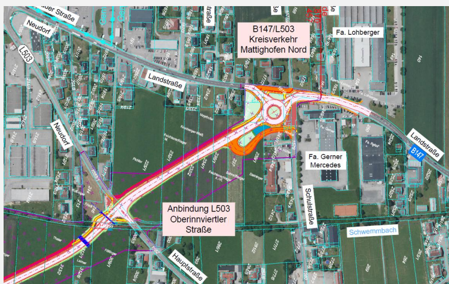
(Abb.: Kreisverkehr "Mattighofen Nord")
