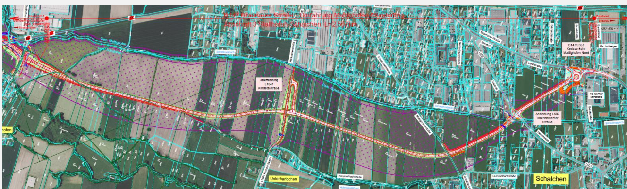
(Abb.: Übersichtslageplan 3. Abschnitt, Stallhofen – Munderfing)
