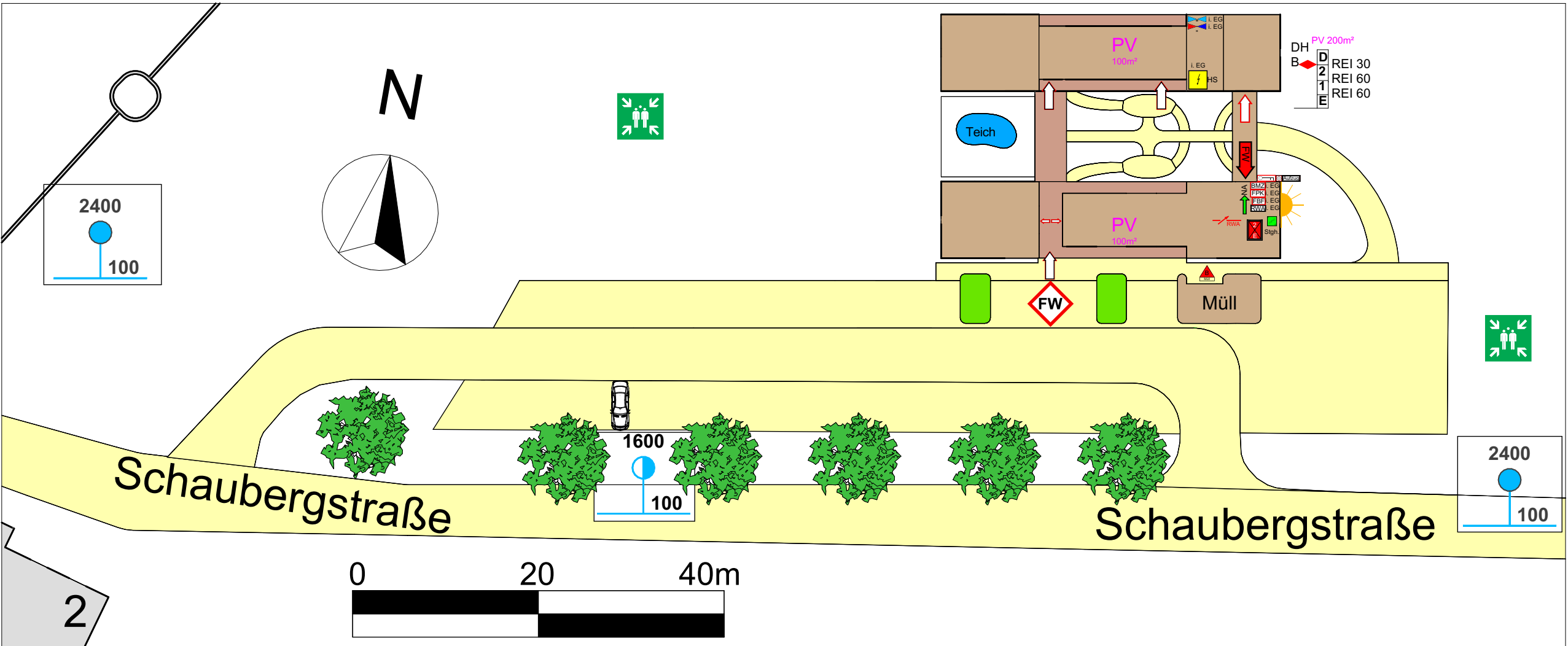
Lageplan-Brandschutz - 1:500
