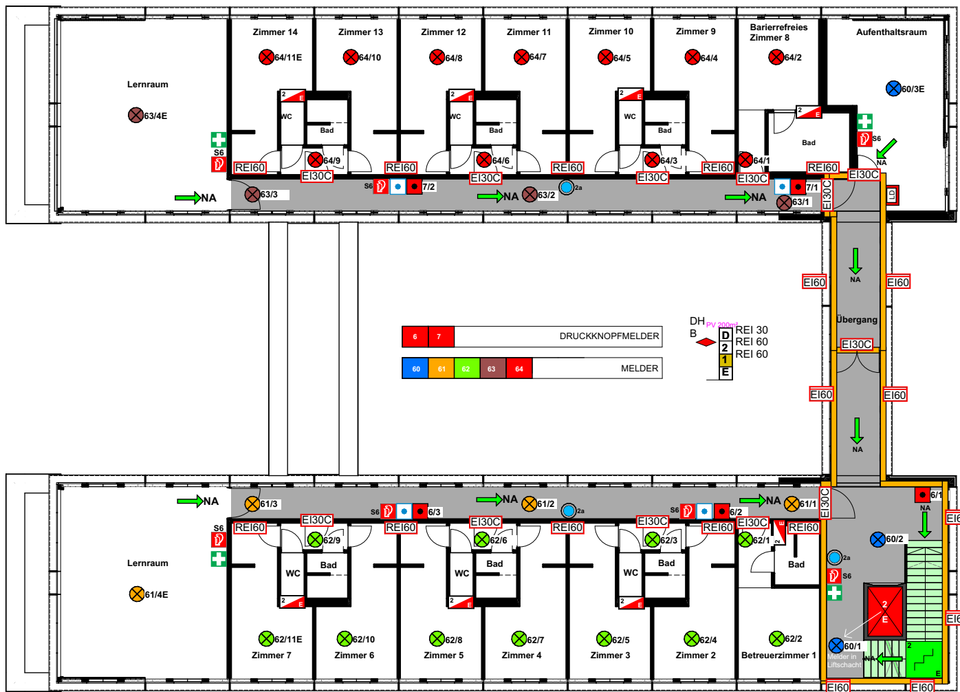
1.OG-Brandschutz - 1:200
