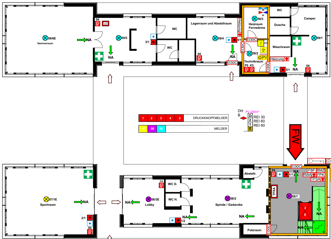
EG-Brandschutz - 1:200
