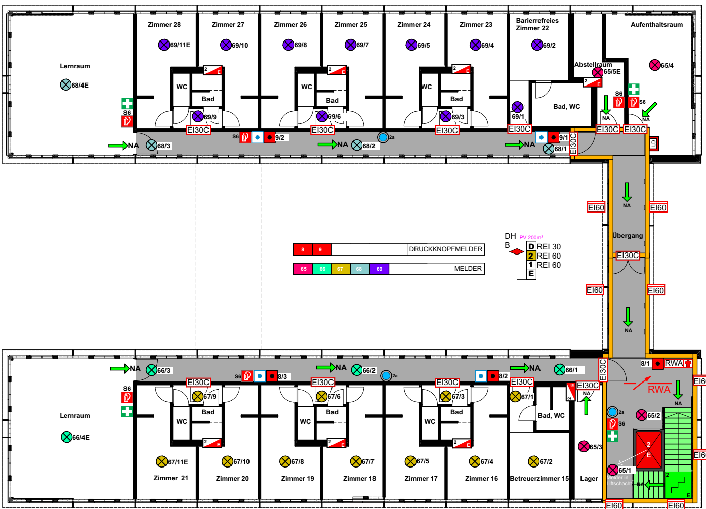
2.OG-Brandschutz - 1:200
