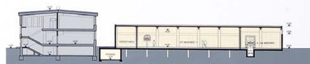
Querschnitt D (Schnitt D)
