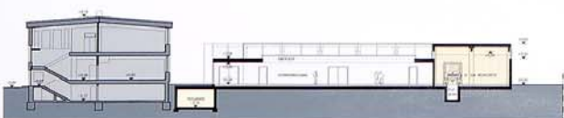
Querschnitt C (Schnitt C)
