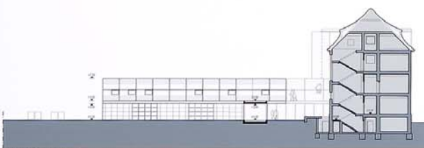
Querschnitt E (Schnitt E)
