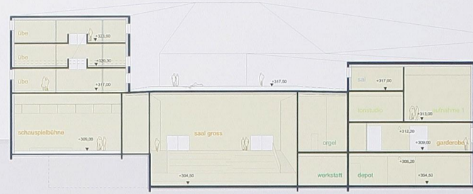
schnitt 3
