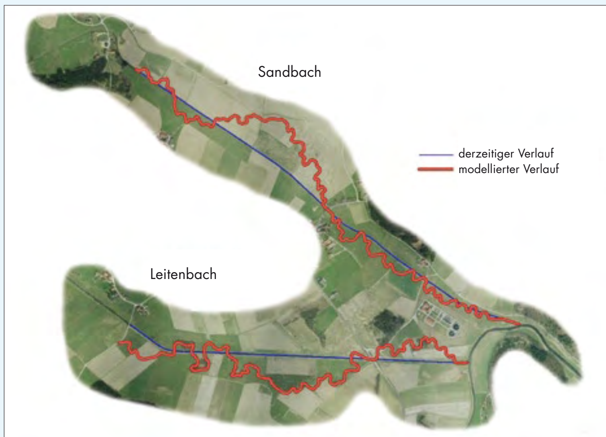
Abb. 48: Gegenüberstellung des derzeitigen Verlaufes von Sandbach und Leitenbach mit dem möglichen Verlauf nach der Renaturierung.
