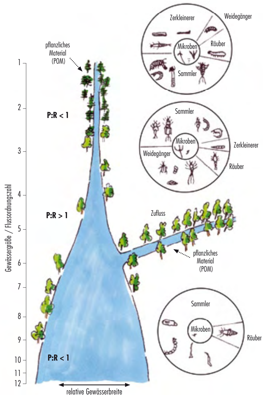
Abb. 27: Schematische Darstellung des Flusslaufes nach dem River-Continuum-Concept (nach VANNOTE et al. 1980). P = Produktion organischen Materials, R = Respiration. POM = partikuläres organisches Material.
