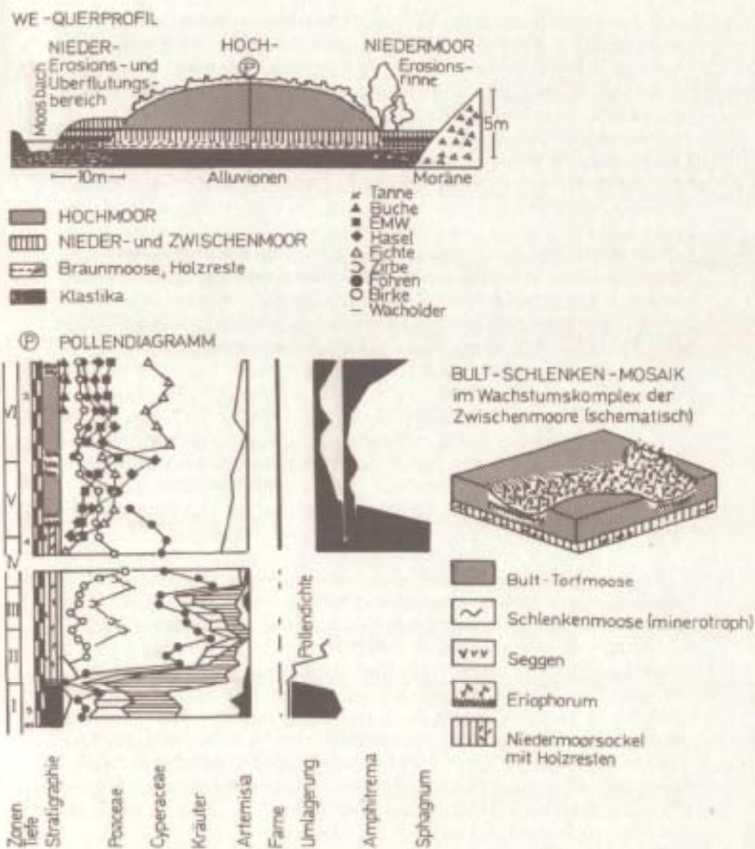
Abbildung 8: Moosalm – Profil, Pollen- und Blockdiagramm.
