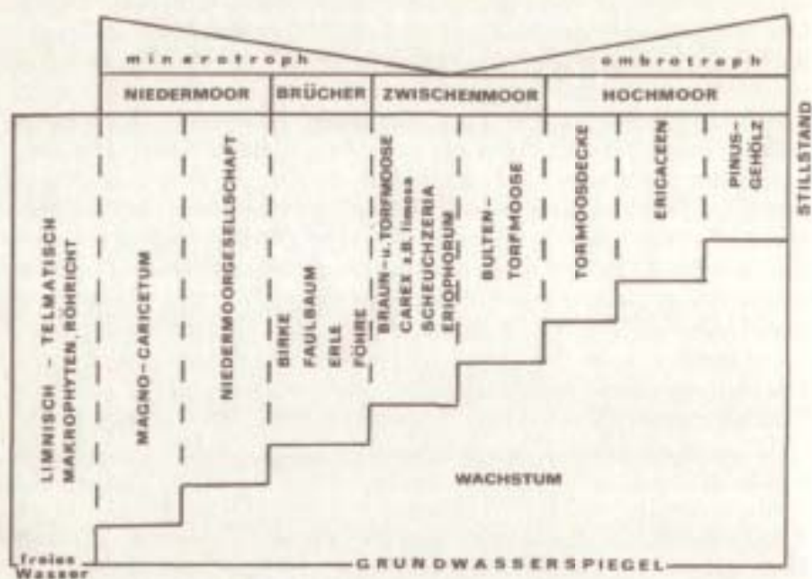
Abbildung 2: Stufen der Moorentwicklung.
