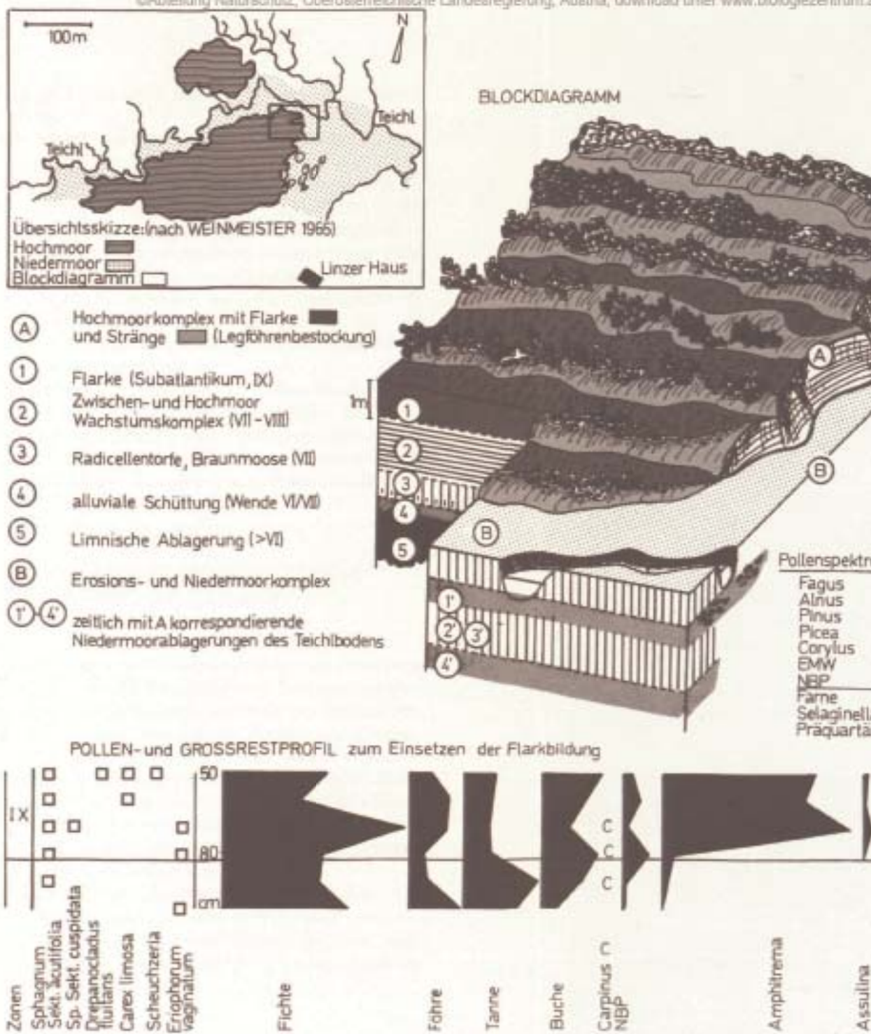
Abbildung 11: Unteres Filzmoos - Profil, Pollen- und Blockdiagramm.
