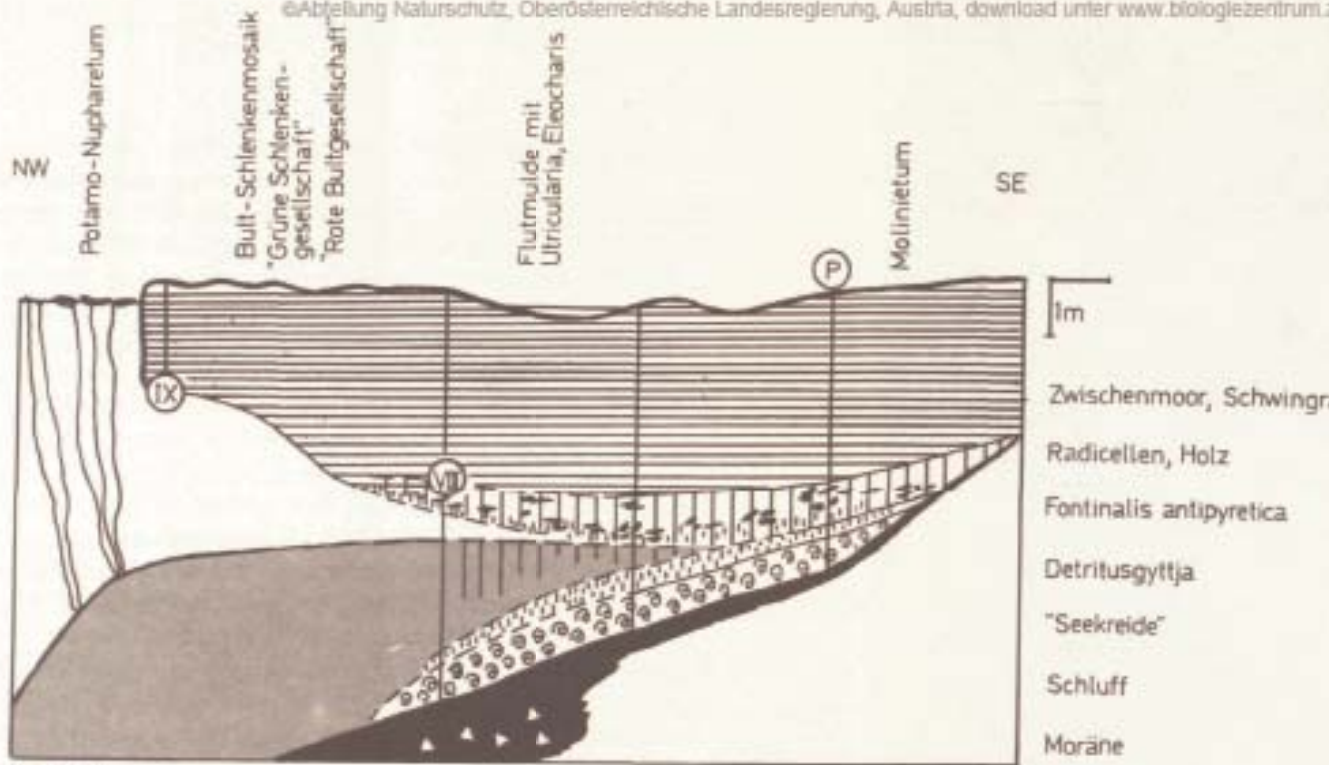
Abbildung 3: Egelsee bei Unterach – Profil und Pollendiagramm.
