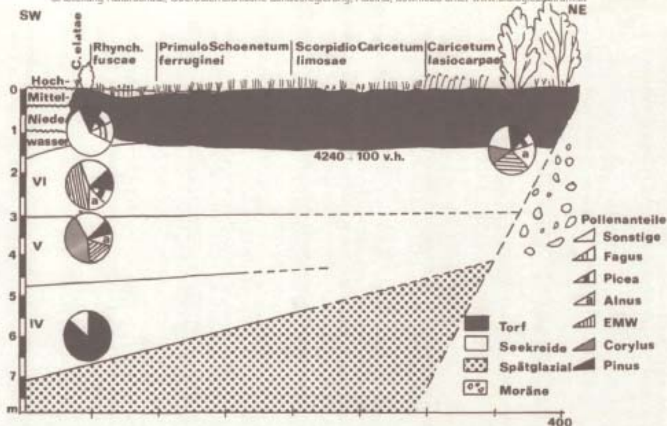
Abbildung 4: Aufbau und Zeitstellung des Niedermoores am Grabensee - NE-Ende. Nach KRISAI 1975.
