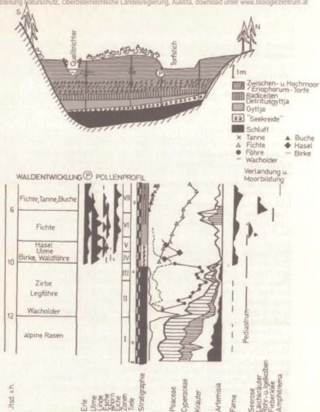
Abbildung 7: Torfmoos/Gosau – Profil und Pollendiagramm.
