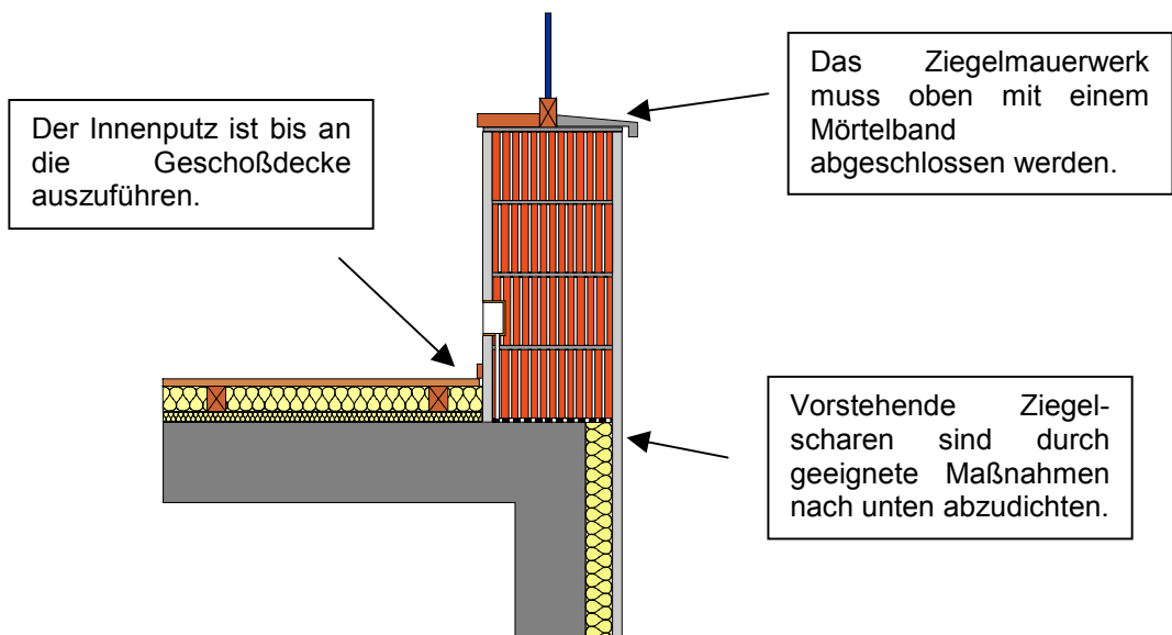
Abb. 8: Ziegelmauerwerk
